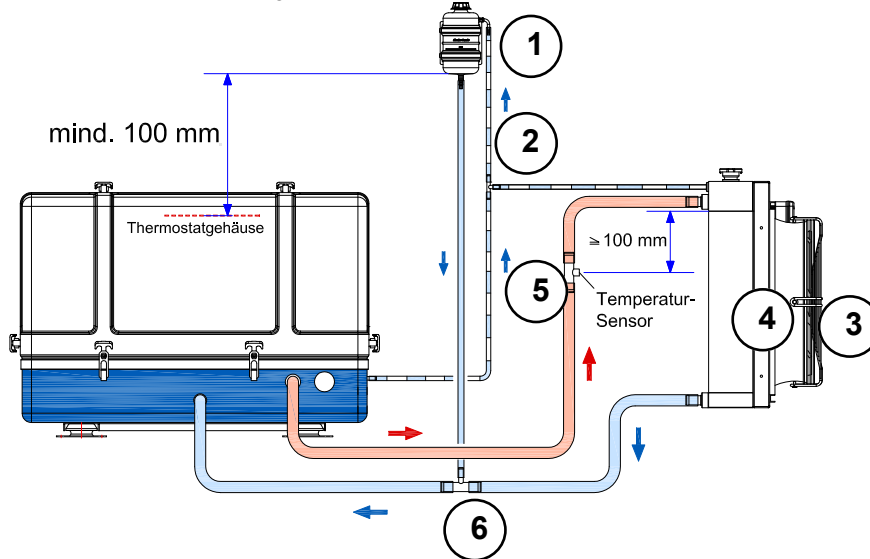
Fig. 5.11.1-1: Vertikaler Kühler - Schema
