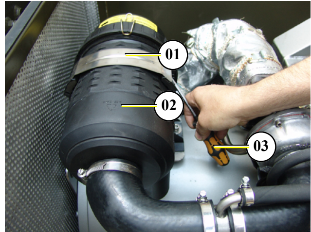
Fig. 7.11-1: Austausch Luftfilter
