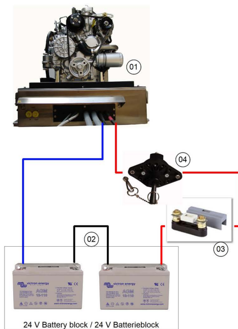
Fig. 5.15.3-2: Starterbatterieanschluss 24 V - Schema
