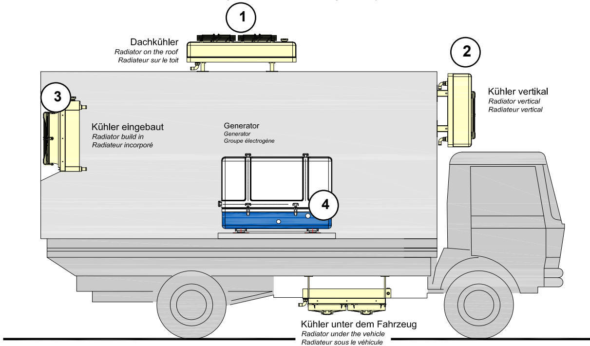
Fig. 5.9.3-1: Kühlermontage - Beispiel
