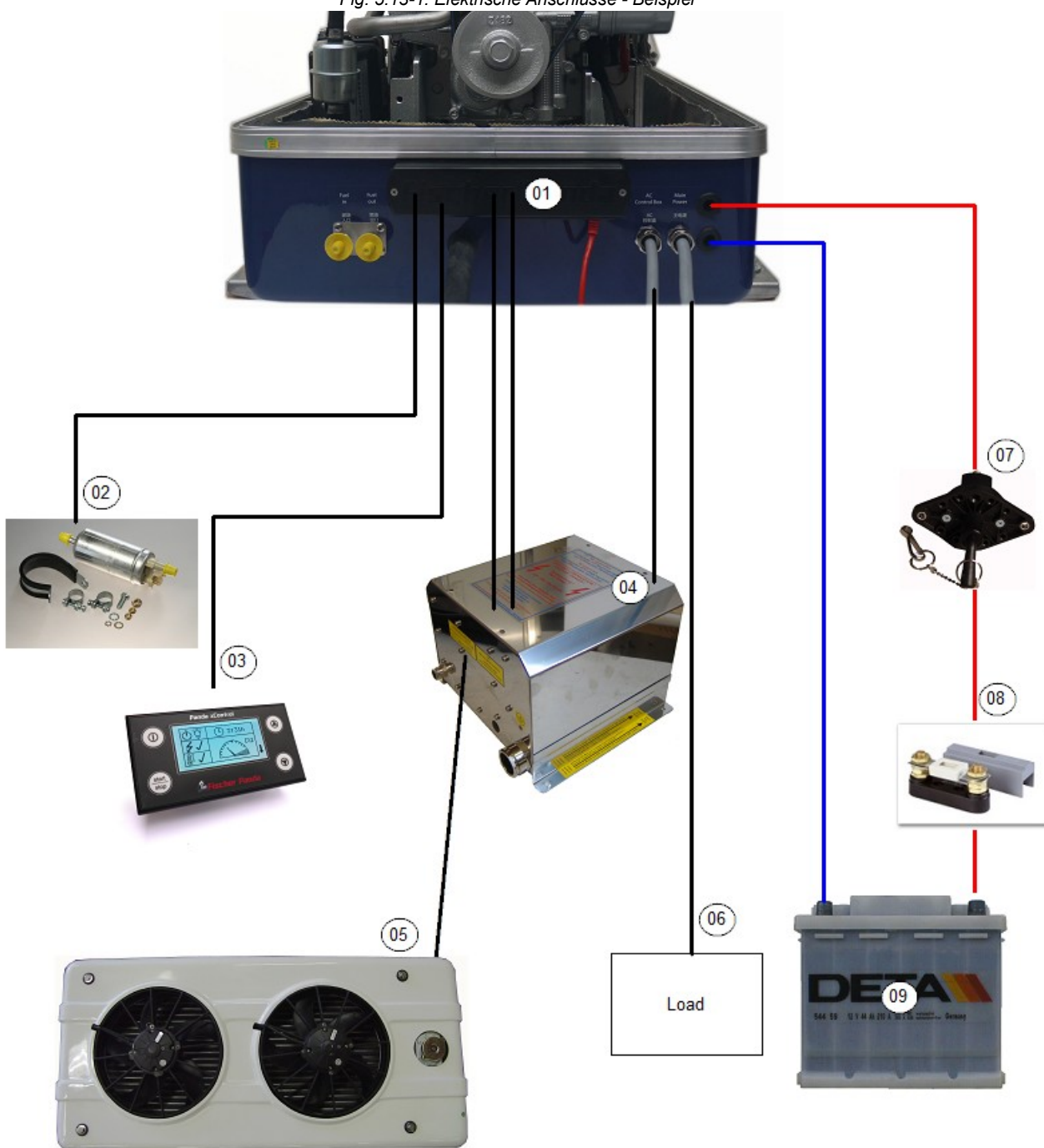
Fig. 5.13-1: Elektrische Anschlüsse - Beispiel
