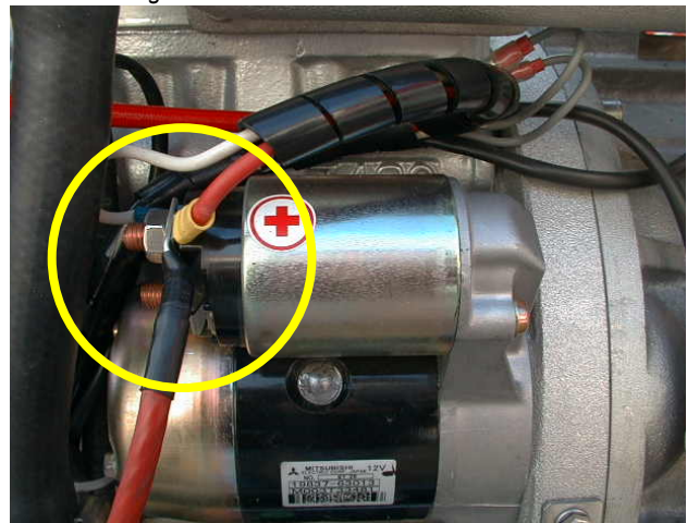
Fig. 5.15.3-4: Pluskabel der Starterbatterie
