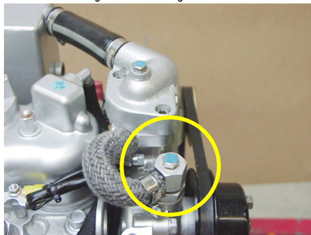
Fig. 7.9-1: Einlüftungsschraube
