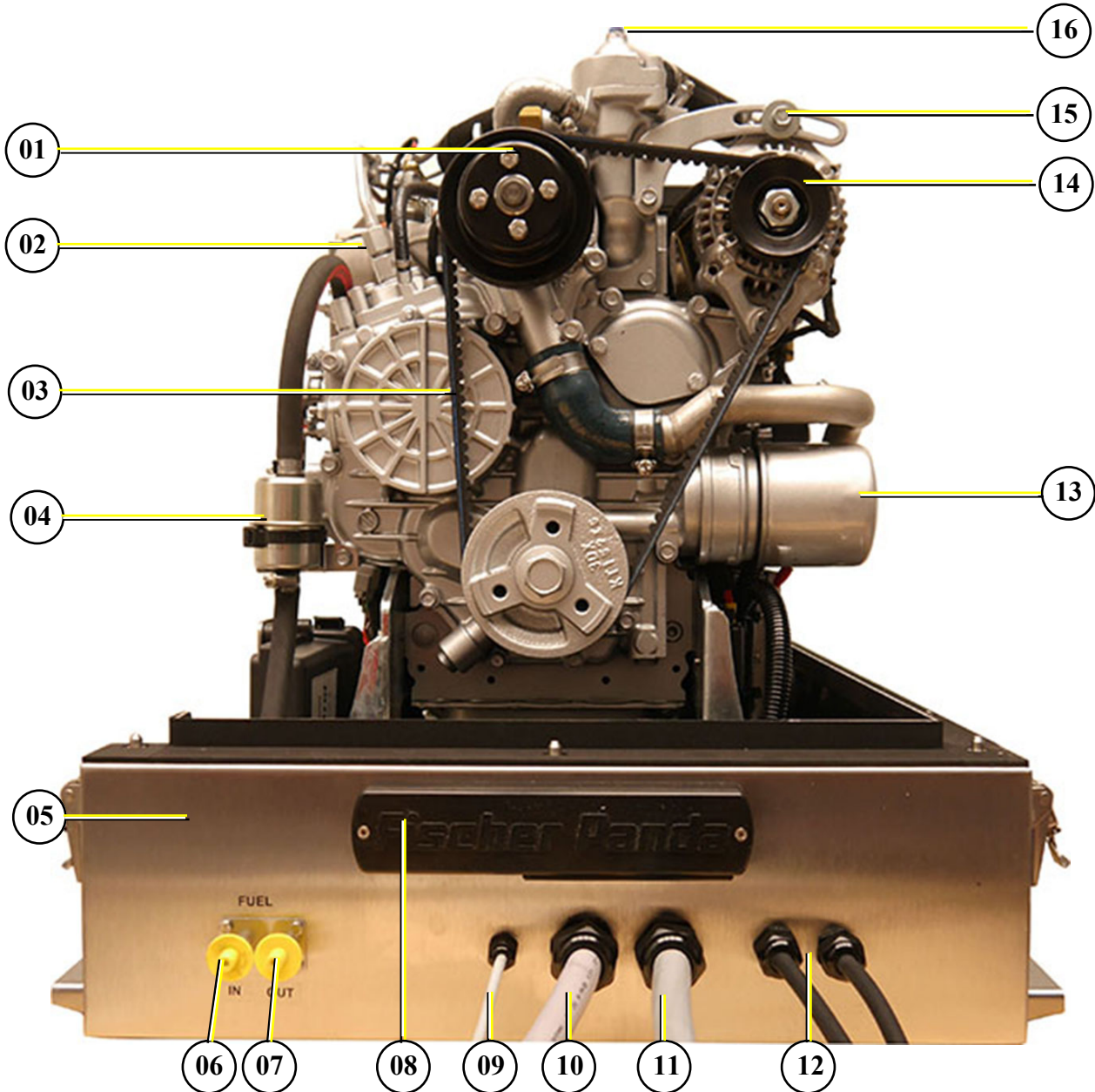
Fig. 4.2.3-1: Seitenansicht Vorderseite
