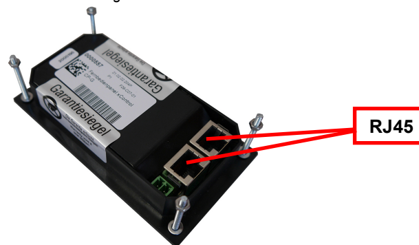
Fig. 2.2-1: xControl CP-G Rückseite
