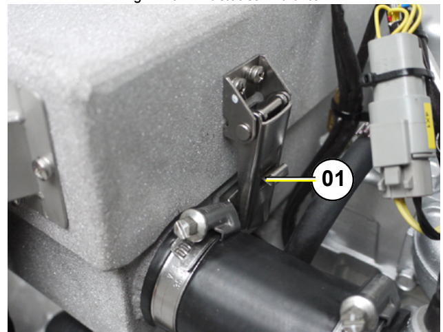
Fig. 7.10-2: Austausch Luftfilter
