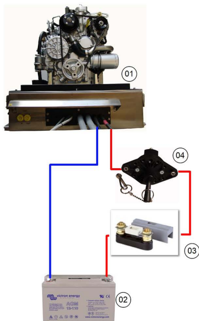
Fig. 5.15.3-1: Starterbatterieanschluss 12 V - Schema
