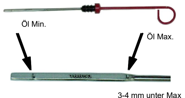
Fig. 7.6.1-1: Ölpeilstab - Beispiel
