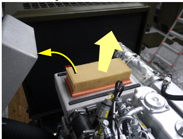
Fig. 7.10-3: Austausch Luftfilter
