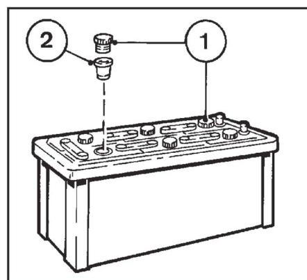
Fig. 7.8.1.2-1: Batterie
