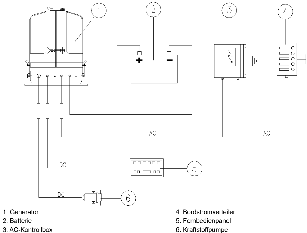
Fig. 5.14.3-1: Installation mit durchgeschliffener AC-Kontrollbox
