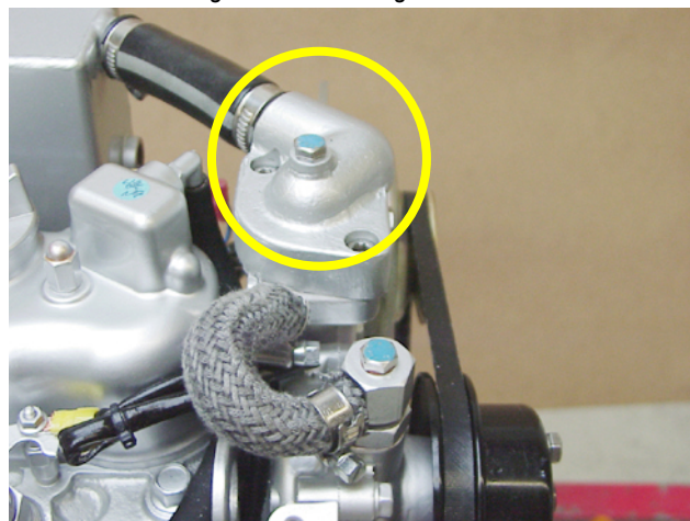
Fig. 7.9-2: Entlüftungsschraube
