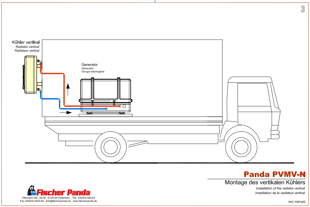
Fig. 5.9.3.3-2: Schema Radiatorkühler Anbau Fahrzeugwand
