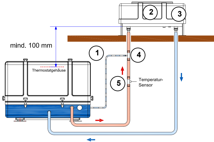
Fig. 5.11.3-1: Dachkühler - Schema
