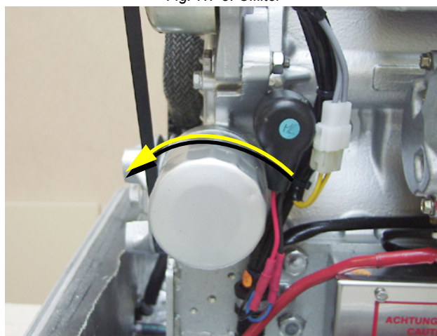
Fig. 7.7-3: Ölfilter
