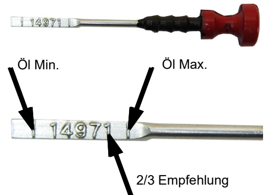
Fig. 7.6.1-2: Beispielbild Ölpeilstab
