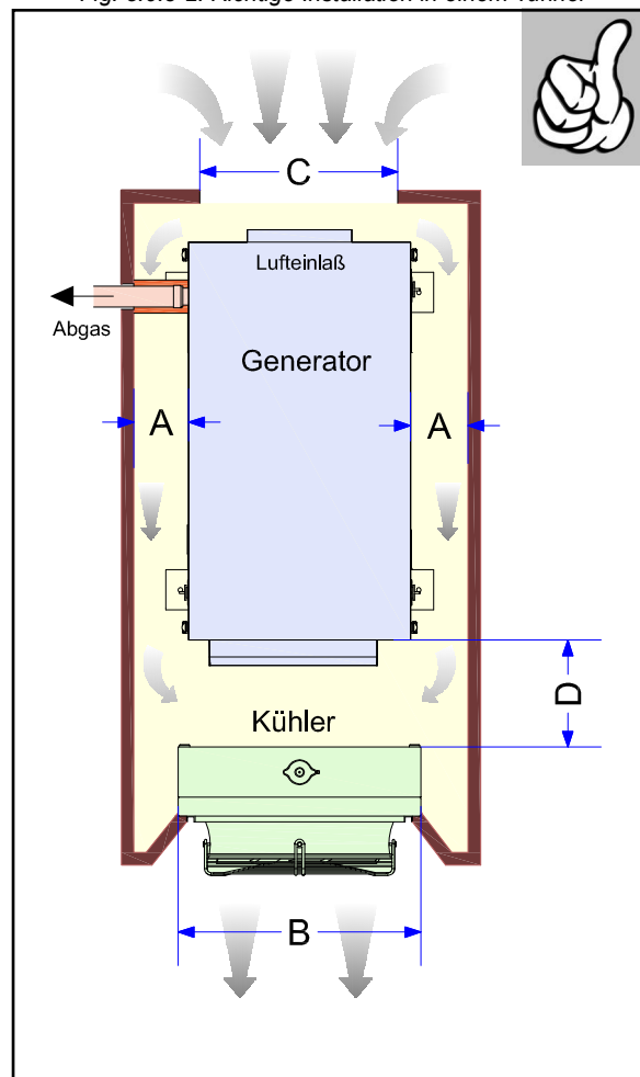
Fig. 5.9.3-2: Richtige Installation in einem Tunnel
