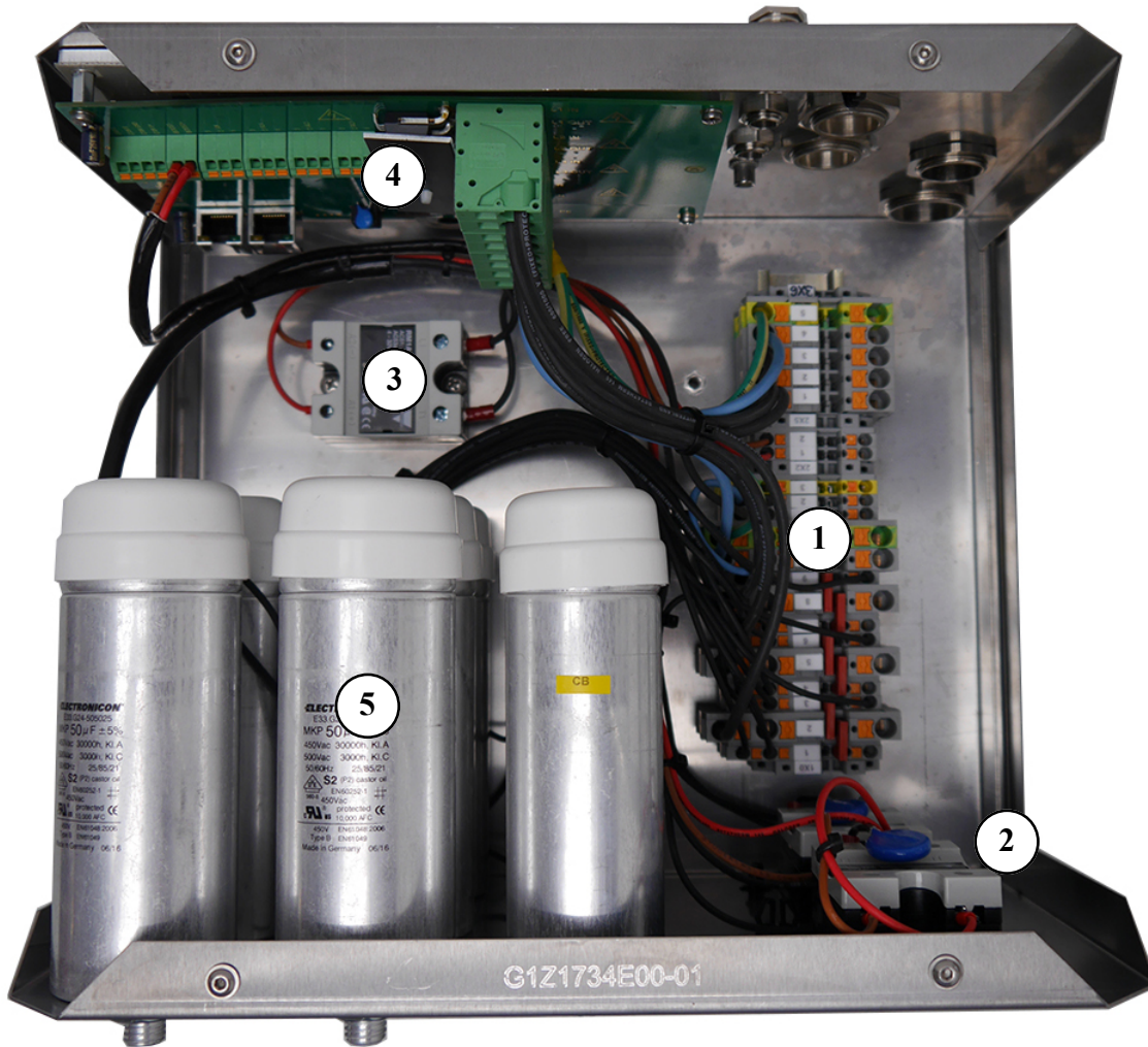
Fig. 5.14.2-2: AC-Kontrollbox dreiphasig - Beispiel
