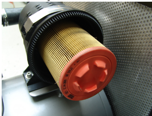
Fig. 7.11-5: Austausch Luftfilter
