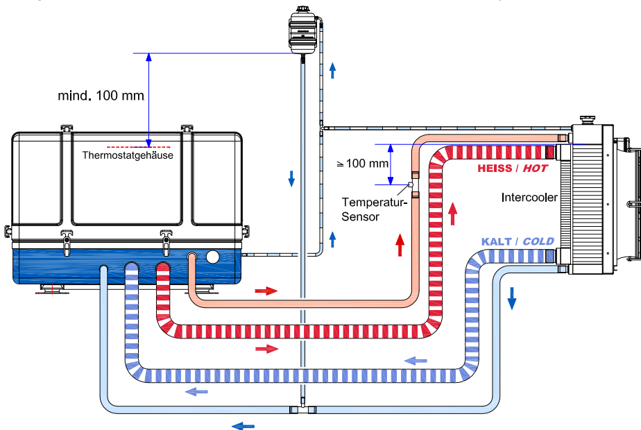
Fig. 5.11.4-1: Installation eines Radiators mit Intercooler - Schema - Beispiel vertikaler Kühler
