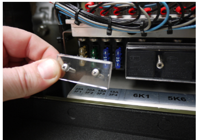
Fig. 7.13-2: Sicherung
