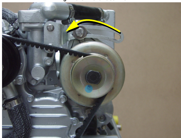
Fig. 7.9-3: Lichtmaschine
