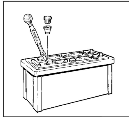
Fig. 7.8.1.3-1: Batterie
