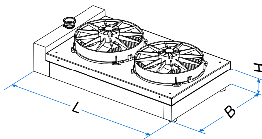
Fig. 5.9.3.1-2: Maße Radiatorkühler
