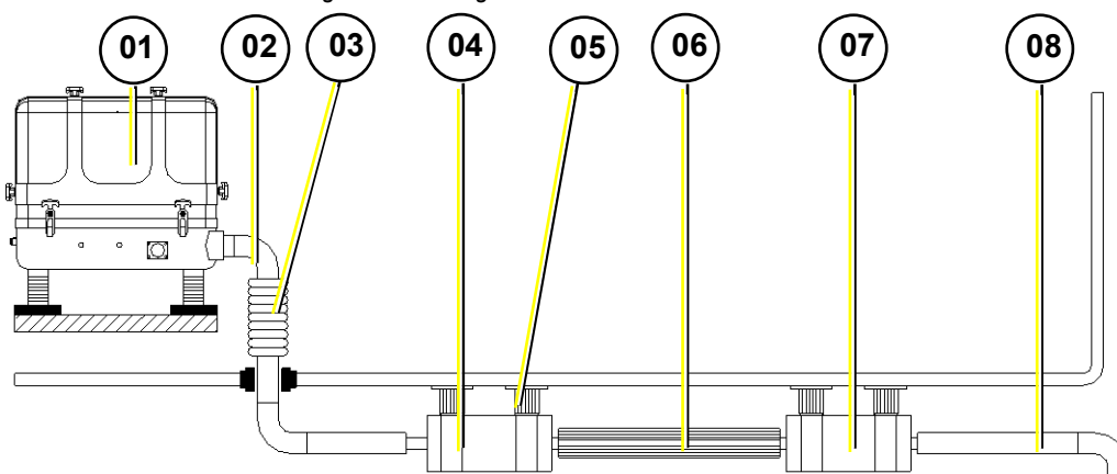
Fig. 5.12.2-1: Abgasinstallation Unterflur - Schema
