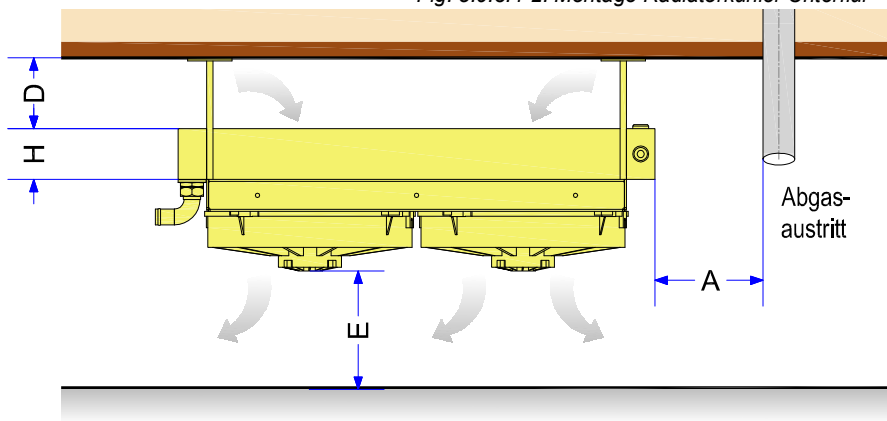
Fig. 5.9.3.4-2: Montage Radiatorkühler Unterflur
