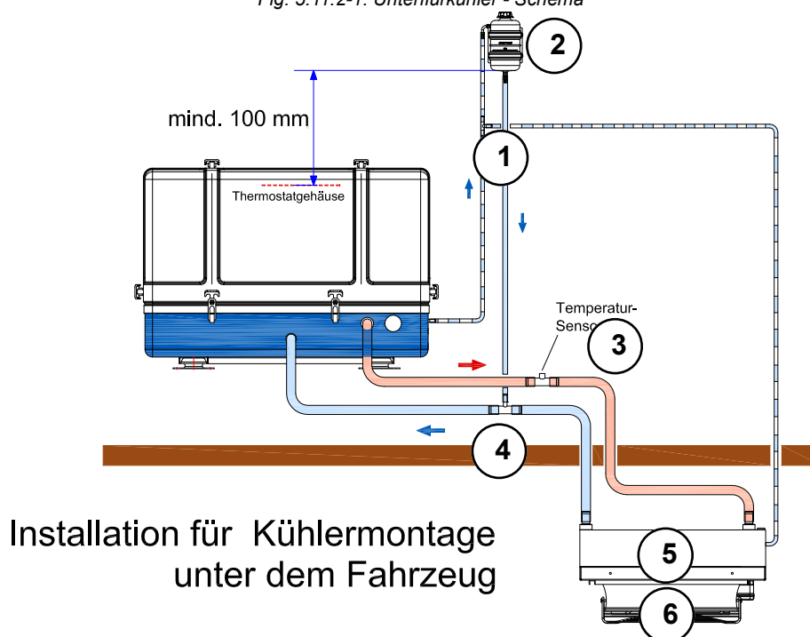
Fig. 5.11.2-1: Unterflurkühler - Schema
