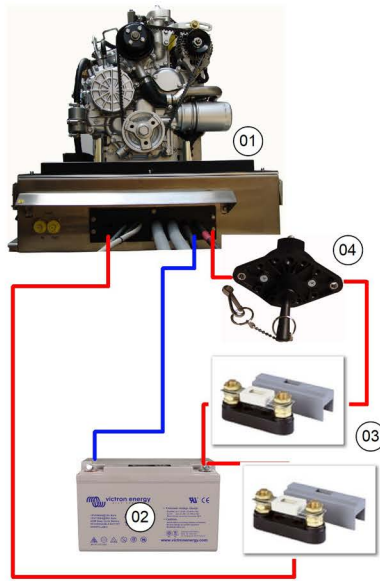
Fig. 5.15.3-3: Starterbatterieanschluss 12 V- Schema mit seperatem Stromanschluss für die ECU
