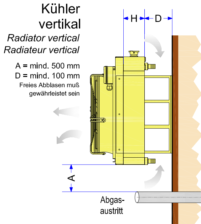
Fig. 5.9.3.3-2: Schema Radiatorkühler Anbau Fahrzeugwand
