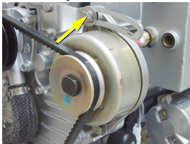
Fig. 7.9-1: Lichtmaschine
