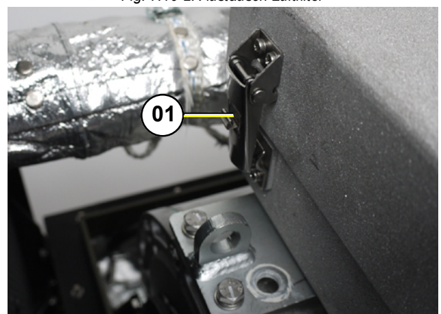
Fig. 7.10-2: Austausch Luftfilter
