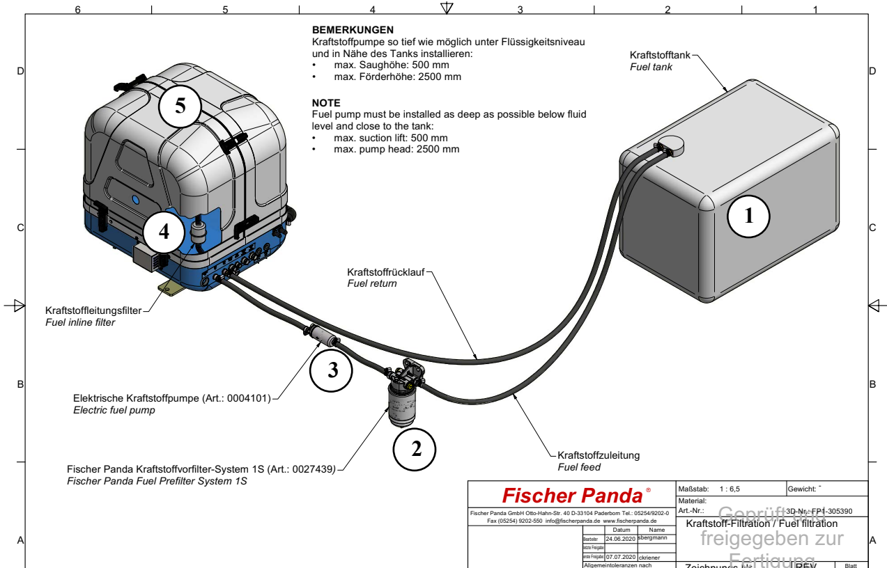
Fig. 5.6.1-2: Kraftstoffanschluss - Schema
