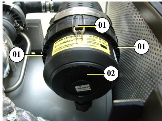
Fig. 7.11-3: Austausch Luftfilter
