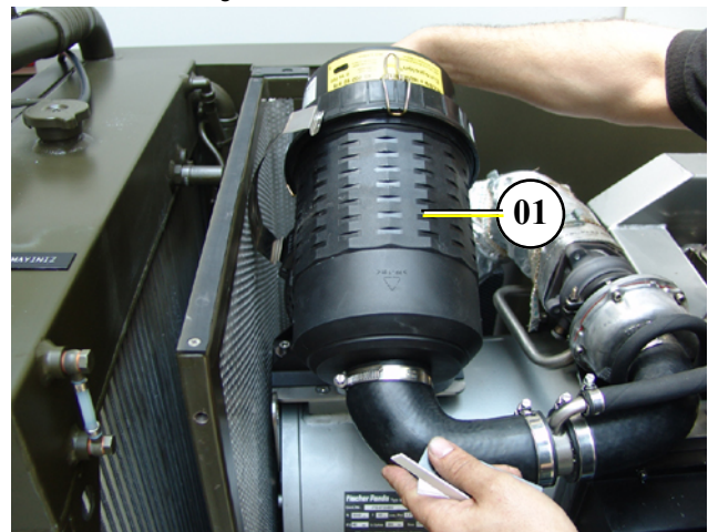
Fig. 7.11-2: Austausch Luftfilter
