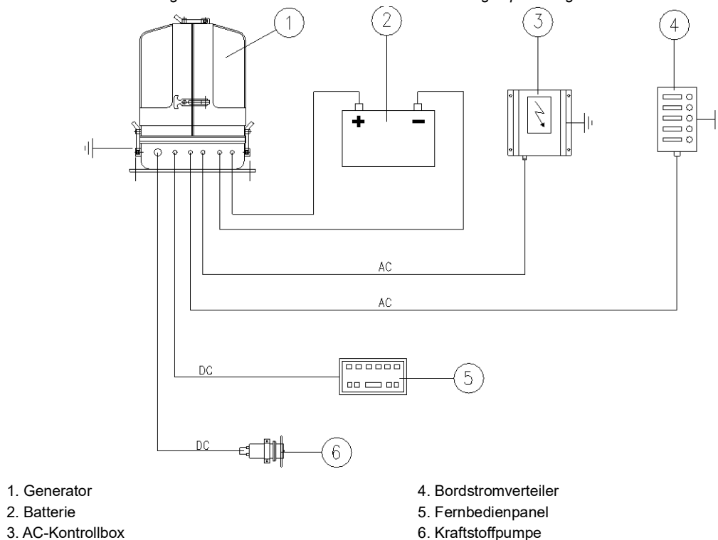
Fig. 5.14.4-1: Installation AC-Box / Bordverteilung separat angeschlossen
