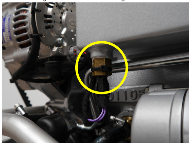
Fig. 4.3.5-2: Thermosensor Abgaskrümmer
