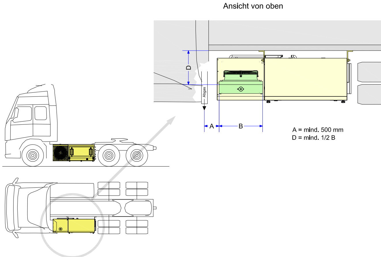
Fig. 5.9.3.7-1: Einbauort PVK-UK
