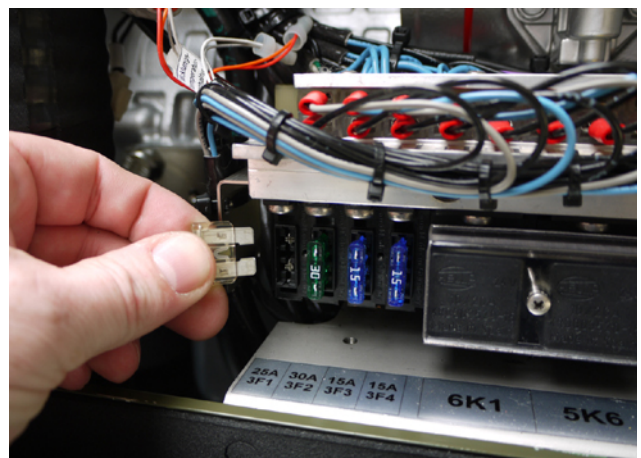
Fig. 7.13-3: Sicherung
