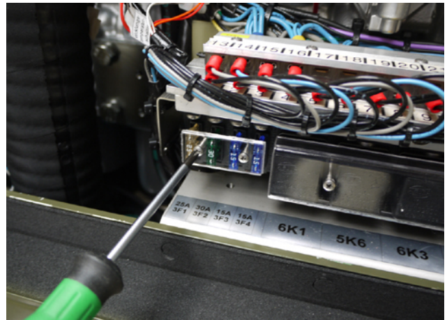
Fig. 7.13-2: Sicherung
