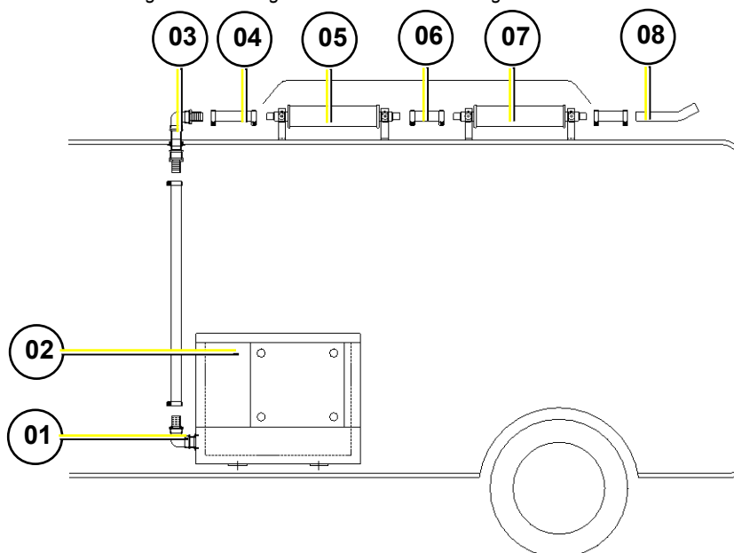
Fig. 5.12.1-1: Abgasinstallation Dachmontage - Schema
