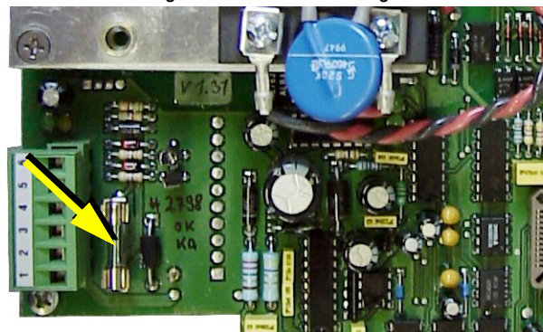
Fig. 8.2.5-1: VCS Sicherung
