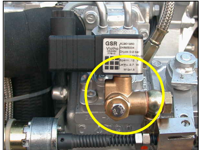
Fig. 5.7.0-1: Entlüftungsschraube am Kraftstoff-Magnetventil
