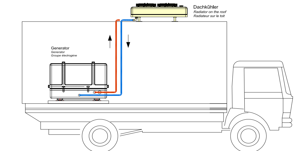
Fig. 5.9.3.2-1: Schema Radiatorkühler Dachaufbau
