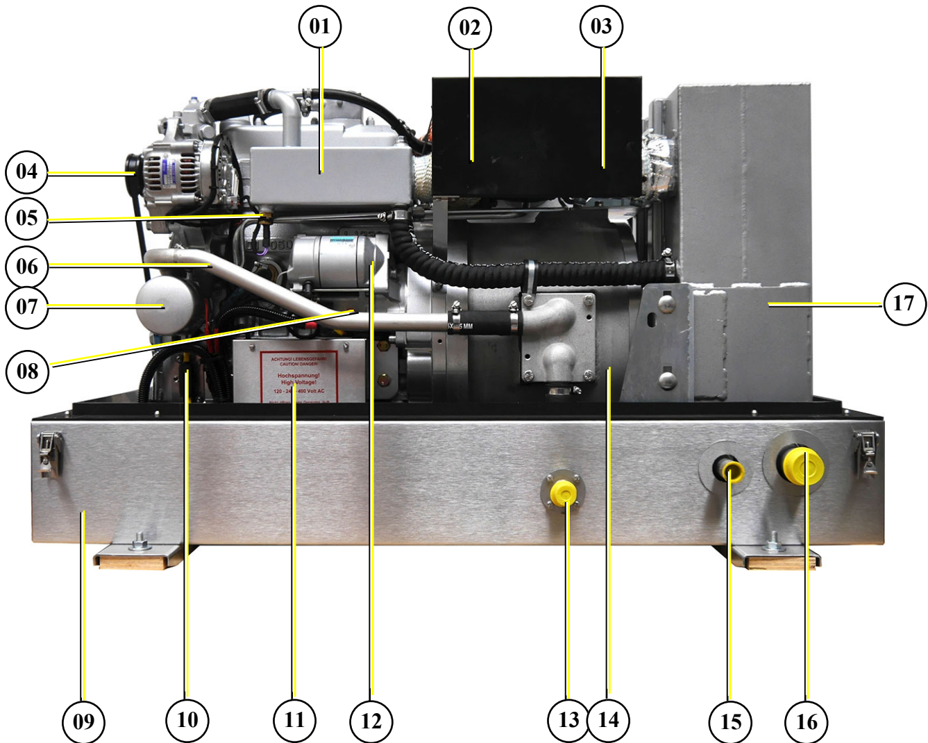
Fig. 4.2.1-1: Seitenansicht Links
