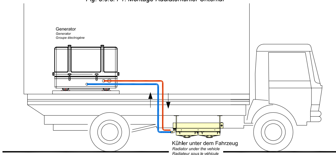
Fig. 5.9.3.4-1: Montage Radiatorkühler Unterflur
