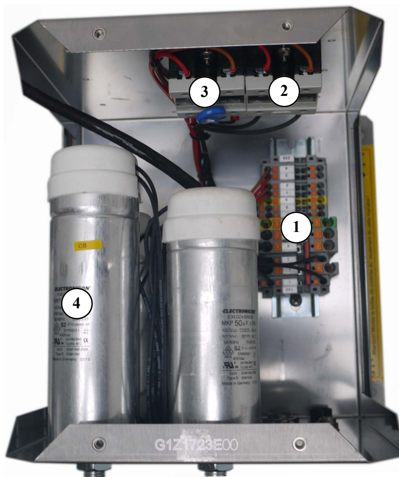
Fig. 5.14.2-1: AC-Kontrollbox einphasig - Beispiel
