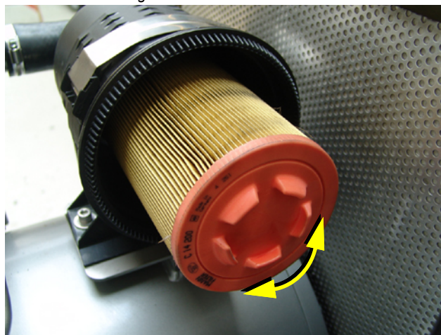
Fig. 7.11-4: Austausch Luftfilter
