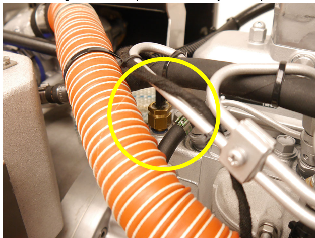
Fig. 4.3.5-1: Temperaturschalter Zylinderkopf
