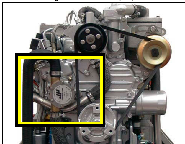
Fig. 10.5.3-3: Gehäuse Seewasserpumpe
