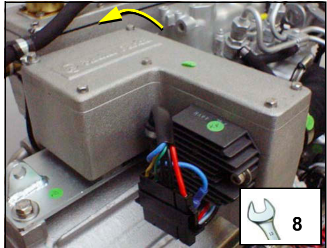
Fig. 10.8.0-1: Luftansauggehäuse
