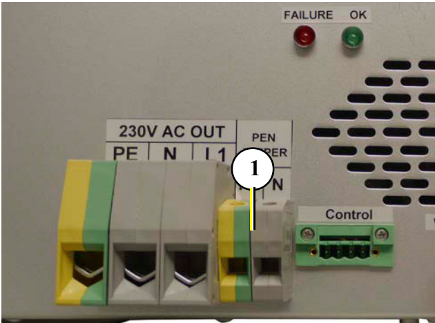
Fig. 20.11-1: PE-N Brücke
