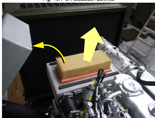
Fig. 10.7-3: Austausch Luftfilter
