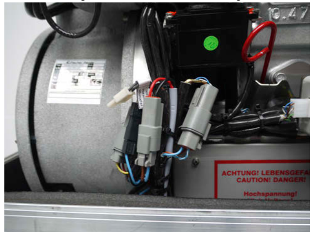
Fig. 7.3.6-3: Thermosensor Wicklung
