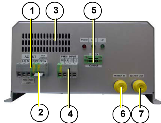
Fig. 20.5-1: Anschlussseite
