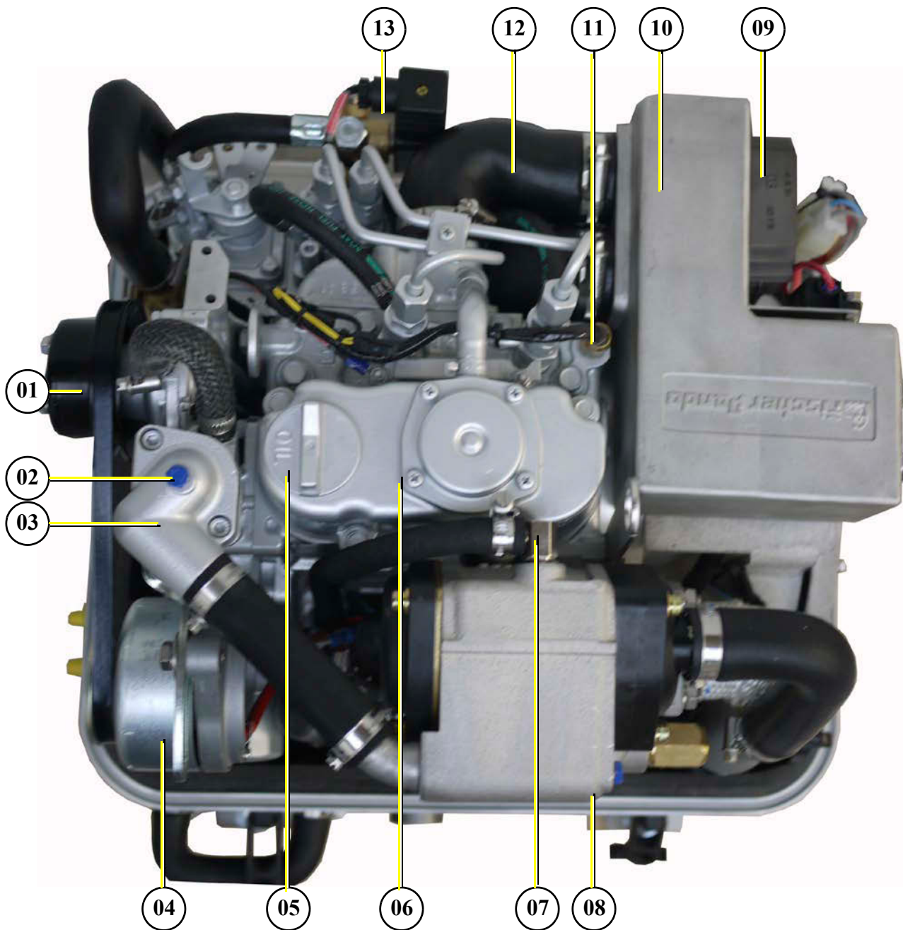
Fig. 7.2.5-1: Draufsicht
