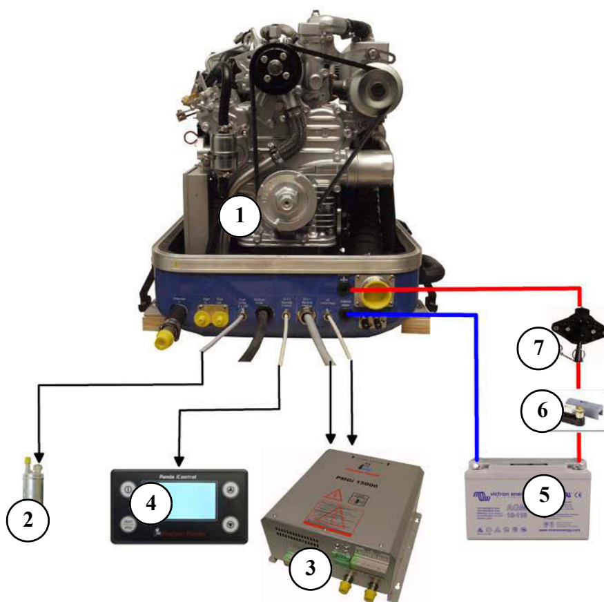
Fig. 8.12.0-1: Installationsschema Beispiel
