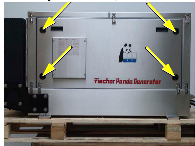
Fig. 5.5-1: Schalldämmkapsel Seitenteil
