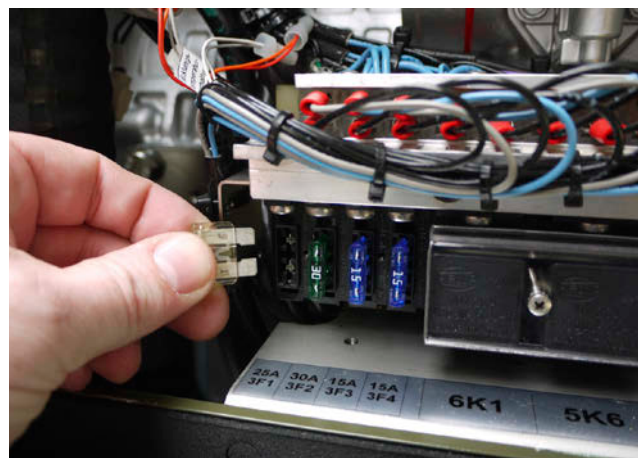
Fig. 10.14-3: Sicherung
