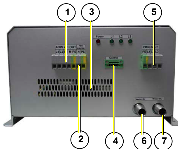
Fig. 20.4-1: Anschlussseite
