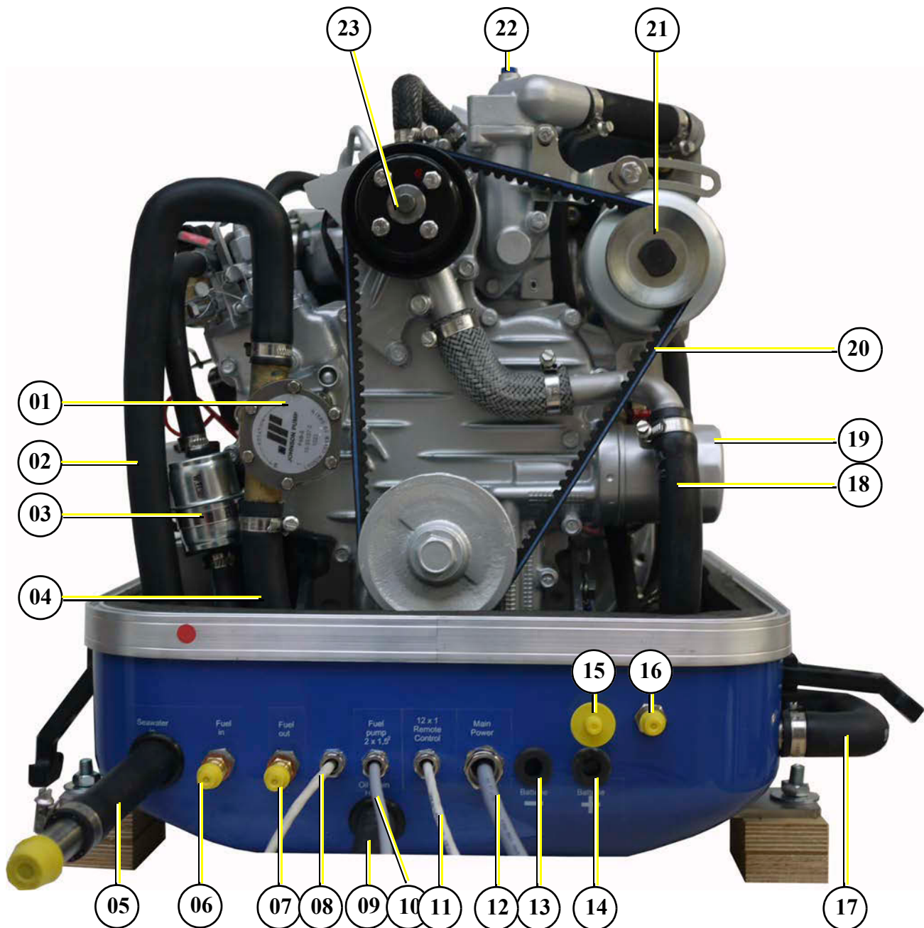
Fig. 7.2.3-1: Vorderansicht
