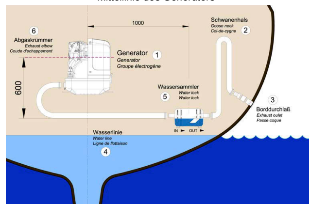
Fig. 8.6.3.2-3: Abgaswassersammler 1000 mm neben der Mittellinie des Generators
