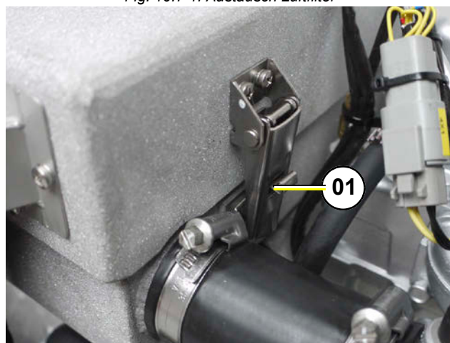
Fig. 10.7-2: Austausch Luftfilter
