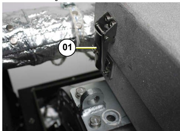
Fig. 10.7-3: Austausch Luftfilter
