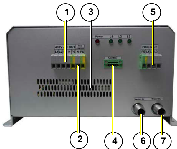
Fig. 19.4-1: Anschlussseite
