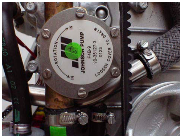
Fig. 9.5.3-3: Gehäuse Seewasserpumpe
