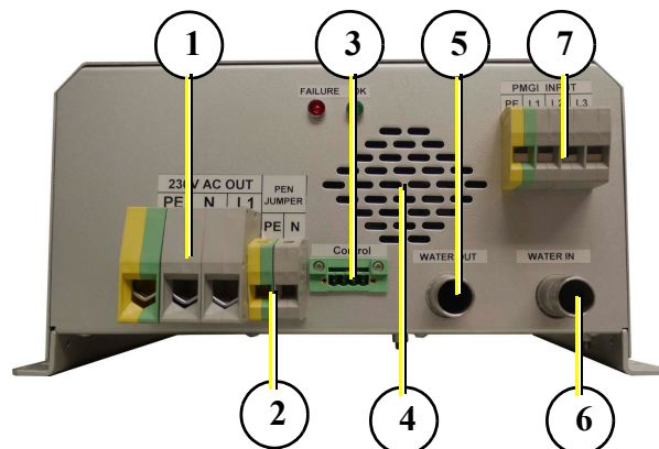
Fig. 19.3-1: Anschlussseite
