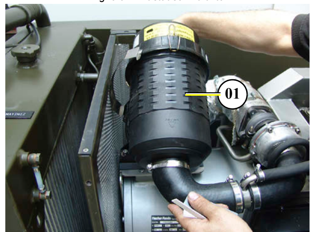
Fig. 9.9-2: Austausch Luftfilter
