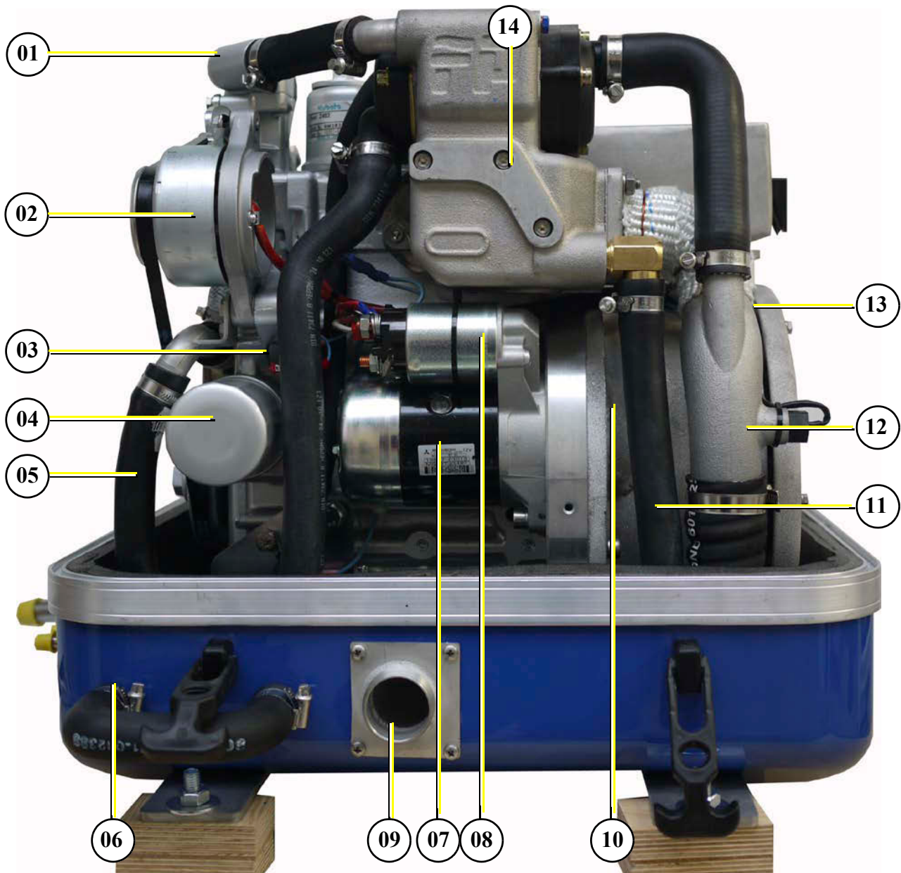
Fig. 6.2.1-1: Seitenansicht Rechts
