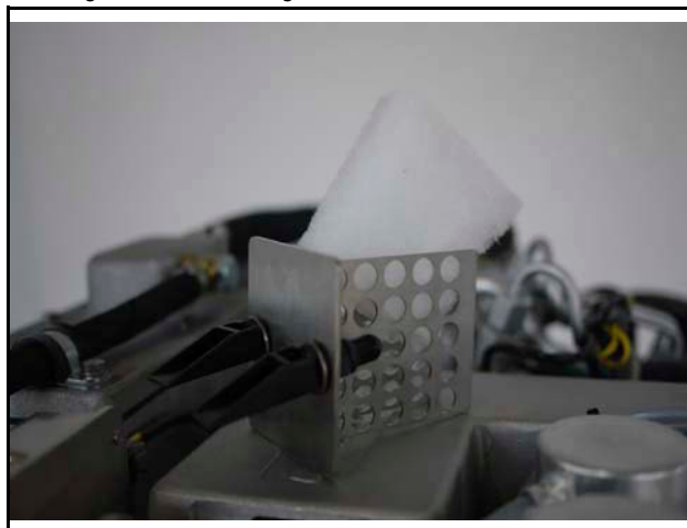
Fig. 9.8.1-4: Luftfiltergehäuse mit Schnellwechselhalter
