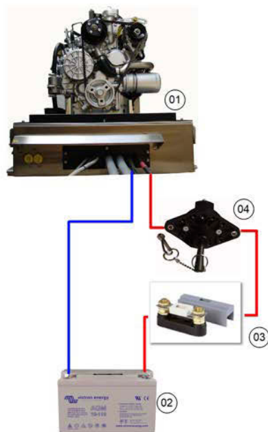
Fig. 7.10.3-1: Starterbatterieanschluss 12 V- Schema
