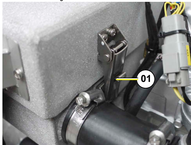
Fig. 9.7-2: Austausch Luftfilter
