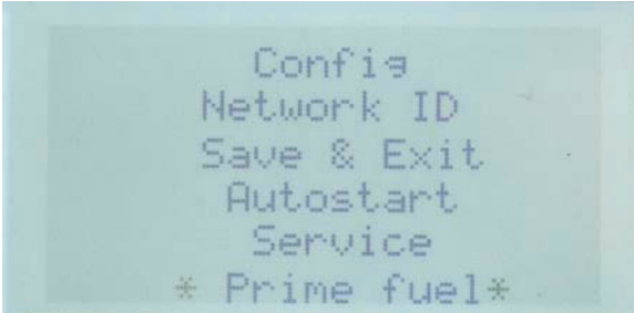
Fig. 14.4.1-2: Setup-Menü
