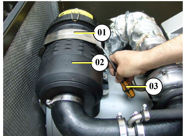
Fig. 9.9-1: Austausch Luftfilter
