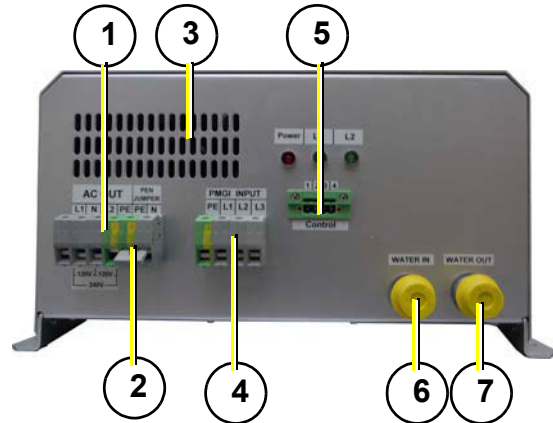
Fig. 19.5-1: Anschlussseite
