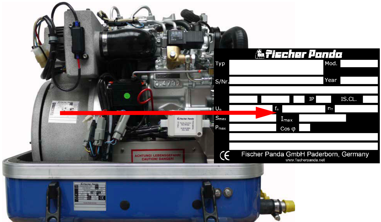
Fig. 6.1-2: Typenschildbeschreibung
