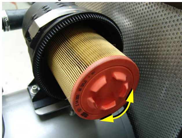
Fig. 9.9-4: Austausch Luftfilter
