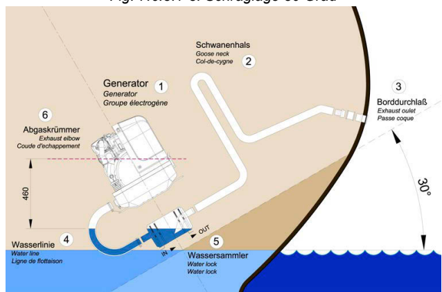
Fig. 7.6.3.1-3: Schräglage 30 Grad
