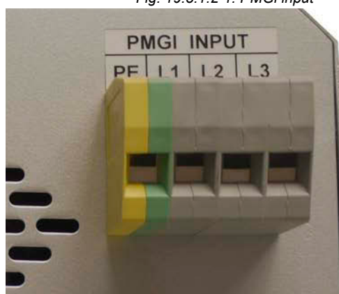
Fig. 19.5.1.2-1: PMGi input
