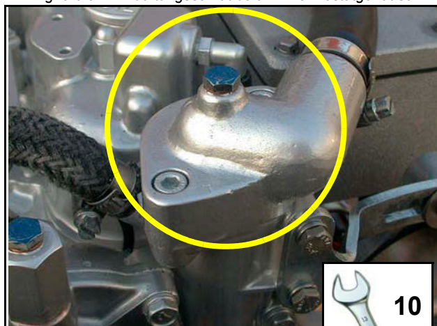
Fig. 9.6.3-2: Entlüftungsschraube am Thermostatgehäuse
