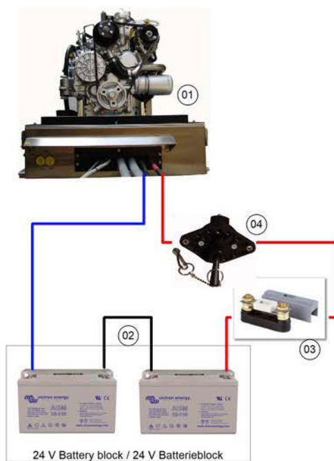
Fig. 7.10.3-2: Starterbatterieanschluss 24 V - Schema
