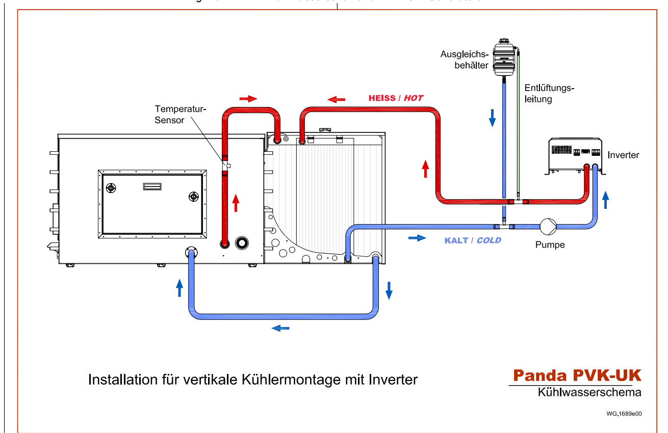
Fig. 19.11.1.2-1: Kühlwasserschema für PVK-UK iGeneratoren
