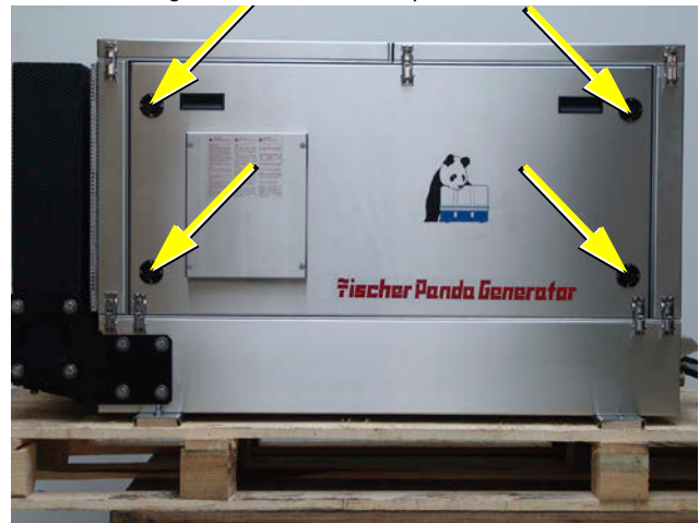
Fig. 4.5-1: Schalldämmkapsel Seitenteil
