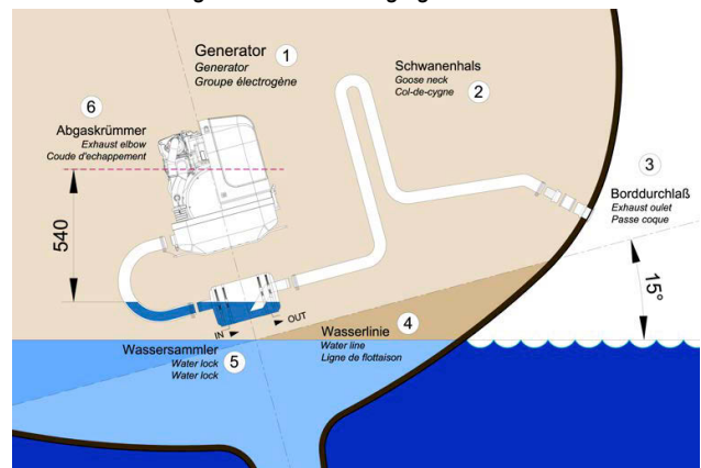
Fig. 7.6.3.1-2: Schräglage 15 Grad
