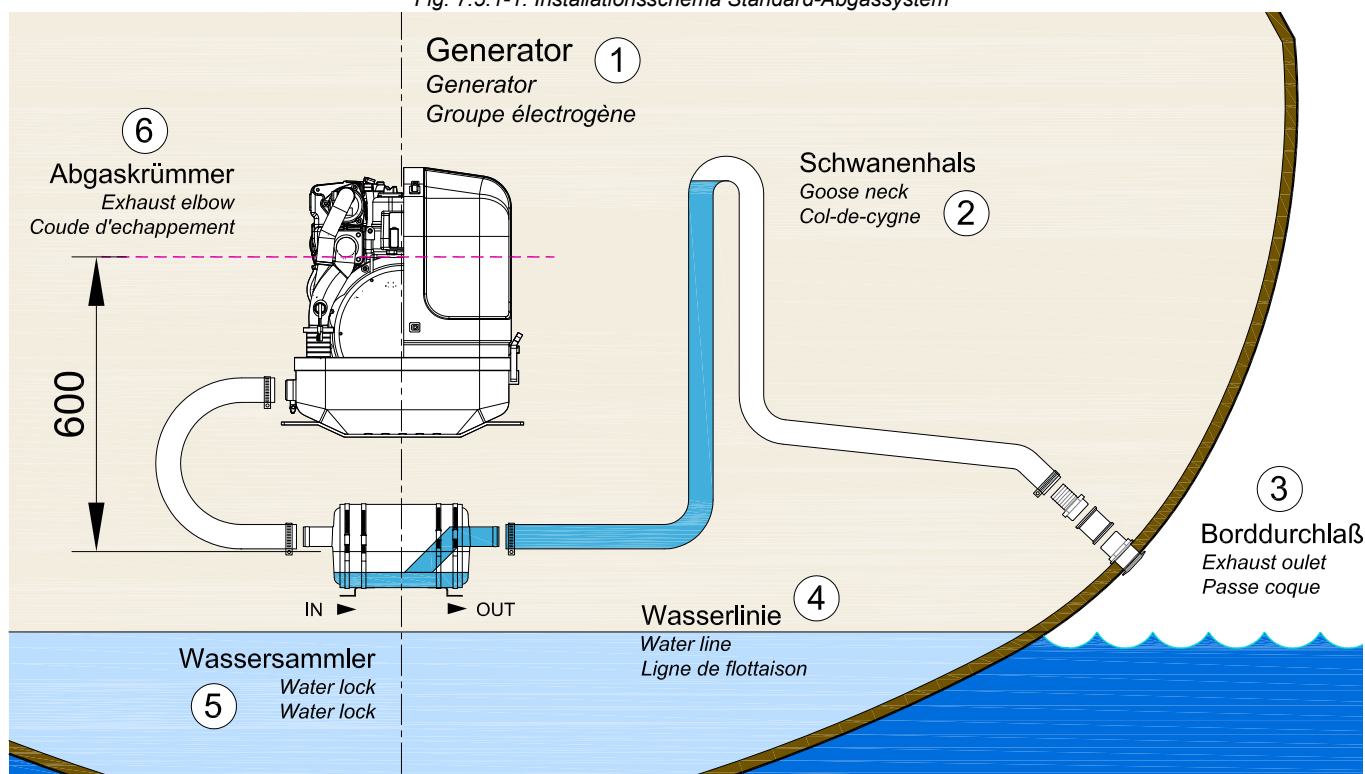
Fig. 7.5.1-1: Installationsschema Standard-Abgassystem
