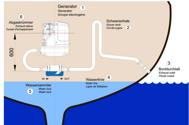
Fig. 7.6.3.1-1: Idealposition des Wassersammlers
