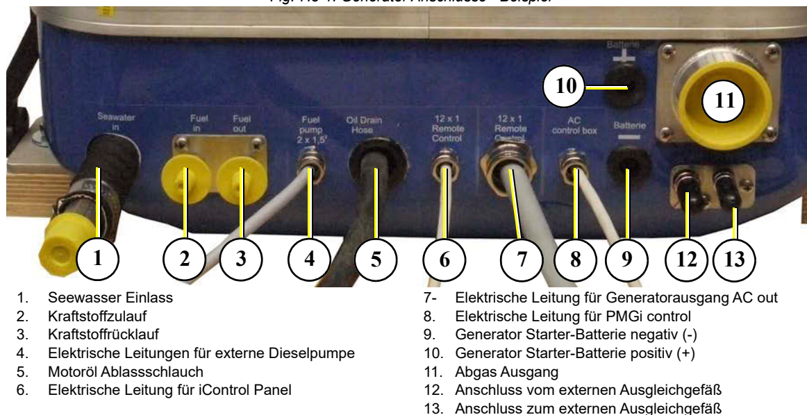
Fig. 7.3-2: Generator Anschlüsse - Beispiel
