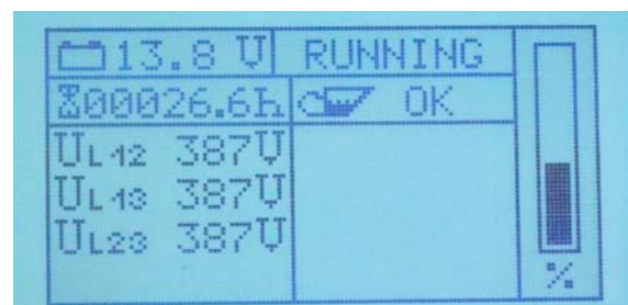
Fig. 14.3.3.4-4: Inverterseite Außenleiterspannungen
