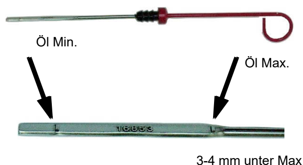
Fig. 9.10.1-1: Ölpeilstab - Beispiel
