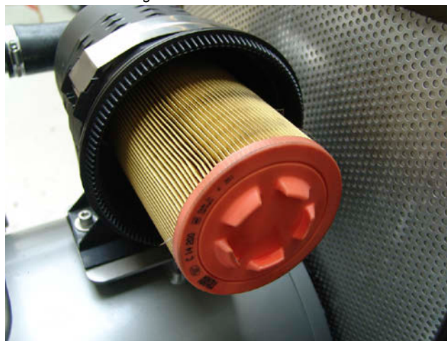
Fig. 9.9-6: Luftfilter reinigen
