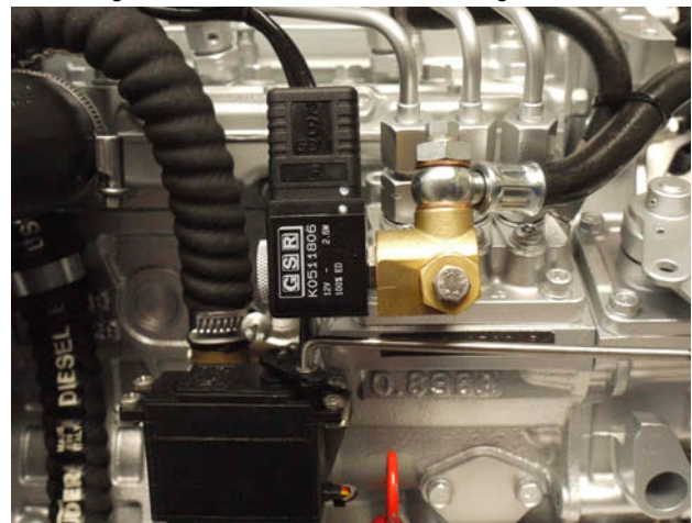
Fig. 10.4.1-1: Elektrisches Kraftstoffmagnetventil
