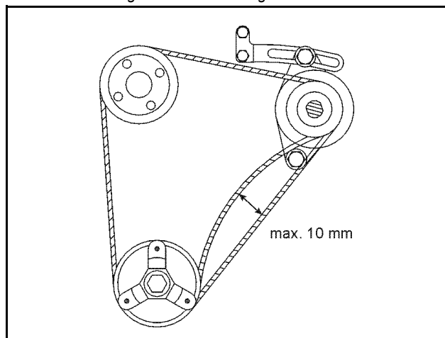
Fig. 9.15-4: Zeichnung Keilriemen
