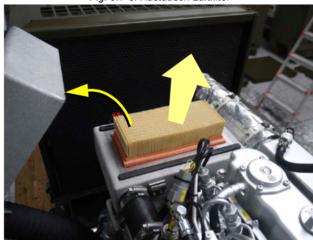
Fig. 9.7-3: Austausch Luftfilter
