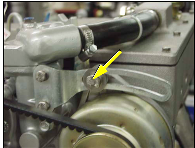
Fig. 9.15-1: Lichtmaschinen-Schraube
