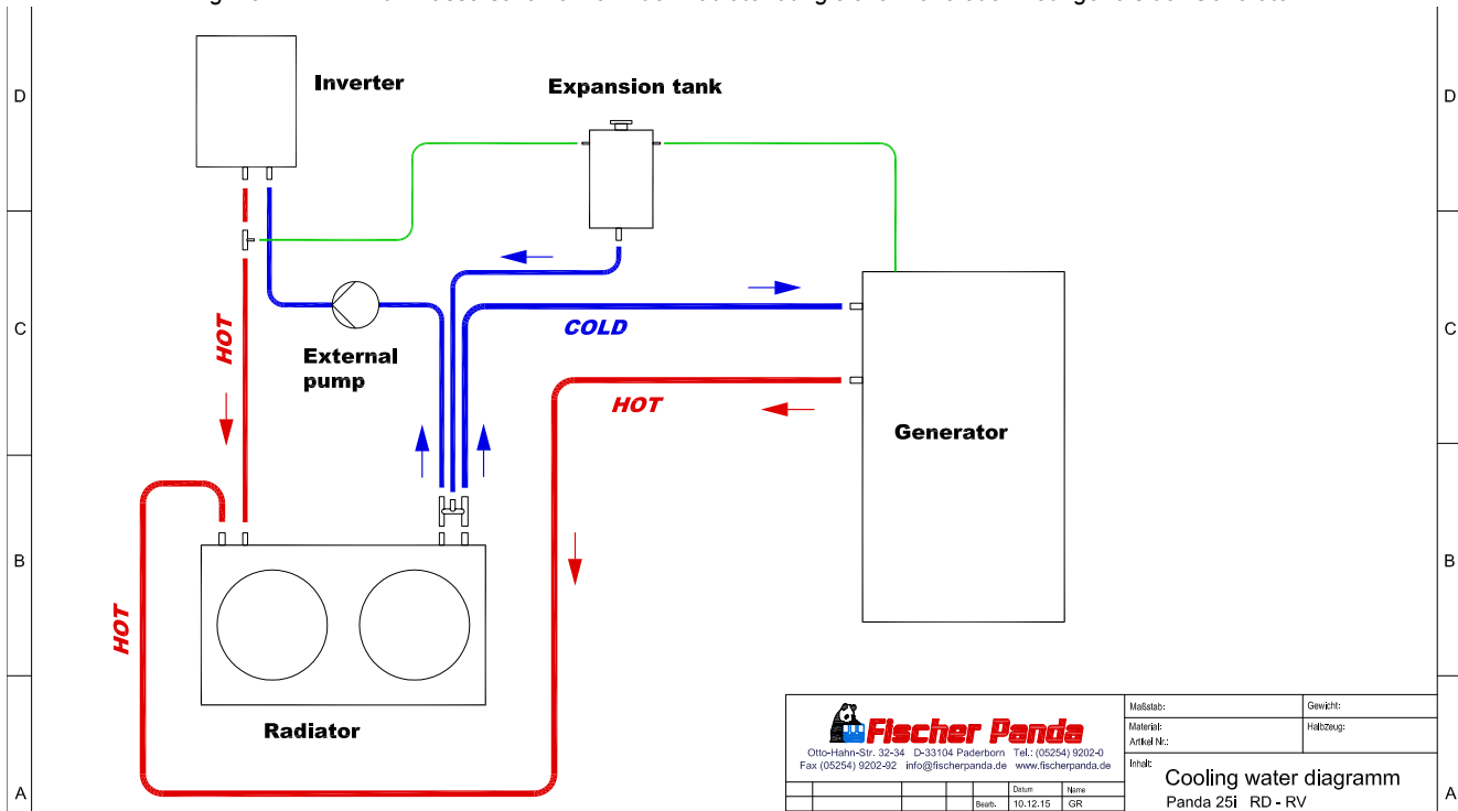
Fig. 19.11.1.1-1: Kühlwasserschema wenn der Radiator auf gleicher höhe oder niedriger als der Generator
