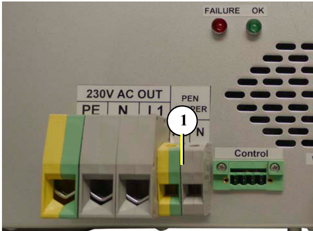
Fig. 19.11-1: PE-N Brücke
