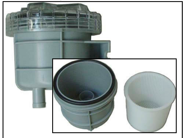
Fig. 9.5.1-1: Seewasserfilter
