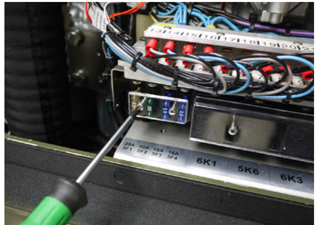
Fig. 9.14-2: Sicherung
