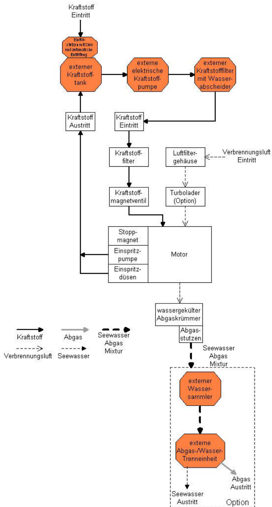
Fig. 6.3.3-1: Kraftstoff-, Verbrennungsluft- und Abgassystem
