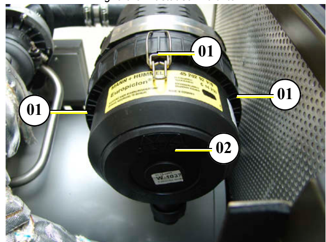
Fig. 9.9-3: Austausch Luftfilter
