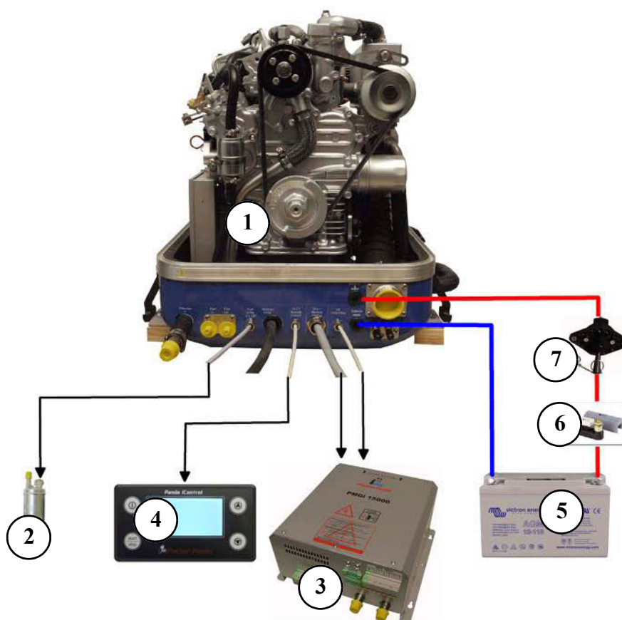
Fig. 7.12.0-1: Installationsschema Beispiel
