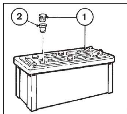
Fig. 9.12.1.2-1: Batterie
