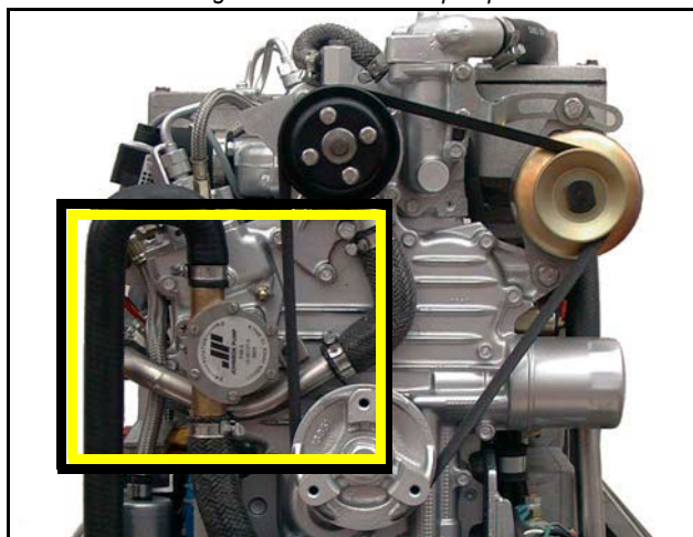
Fig. 9.5.3-3: Gehäuse Seewasserpumpe
