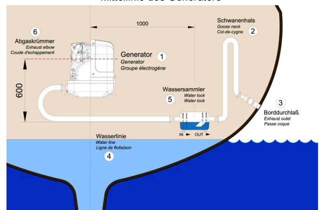
Fig. 7.6.3.2-3: Abgaswassersammler 1000 mm neben der Mittellinie des Generators
