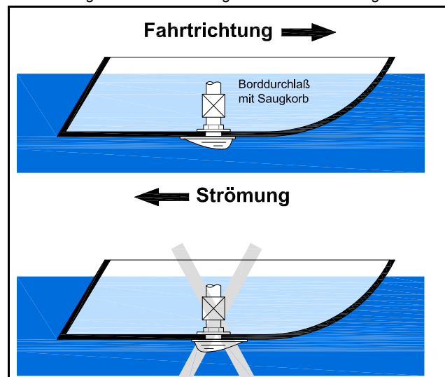
Fig. 7.4.2-1: Anordnung der Borddurchführung
