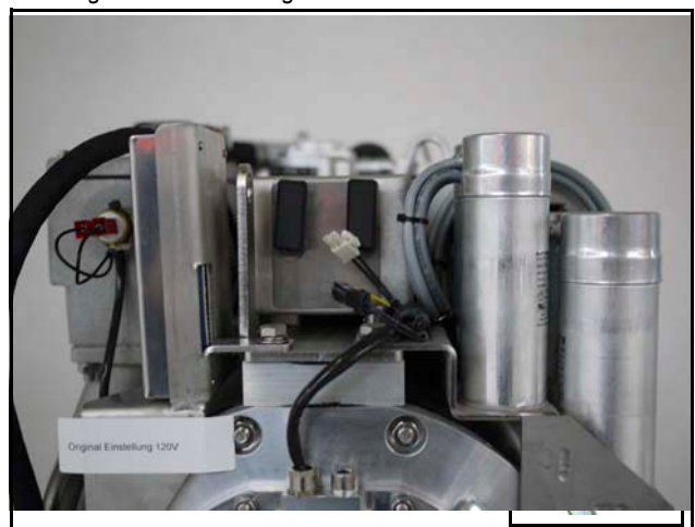
Fig. 9.8.1-1: Luftfiltergehäuse mit Schnellwechselhalter
