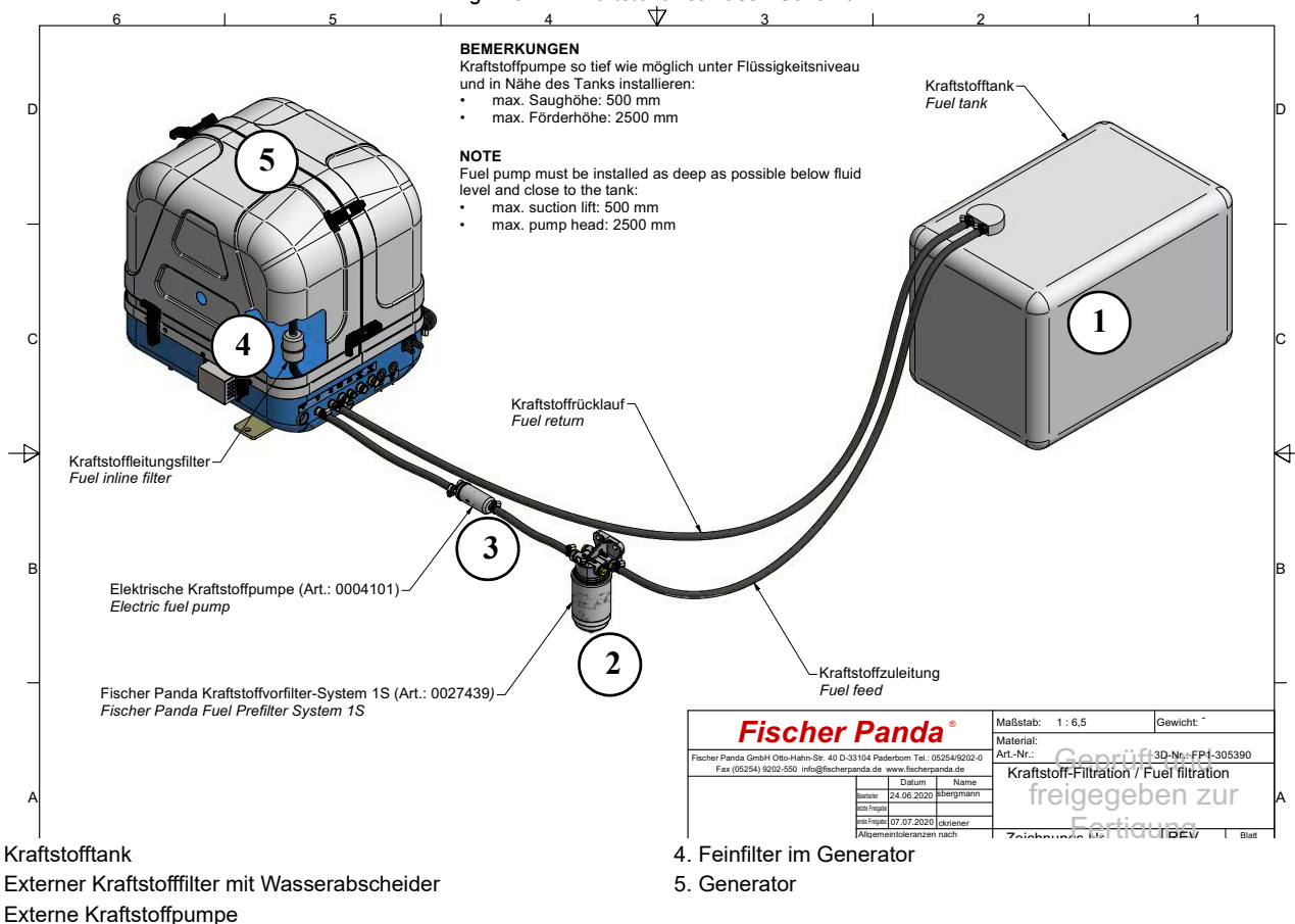
Fig. 7.9.1-2: Kraftstoffanschluss - Schema
