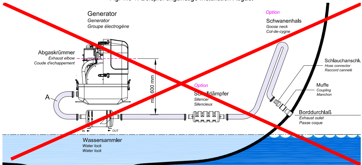
Fig. 7.8-1: Beispiel ungünstige Installation Abgas
