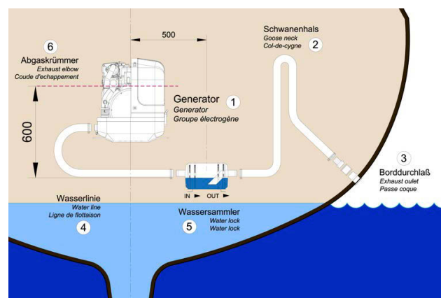
Fig. 7.6.3.2-1: Wassersammler 500 mm neben der Mittellinie des Generators
