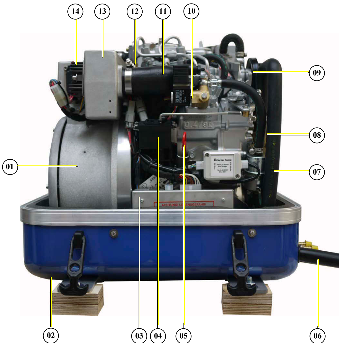
Fig. 6.2.2-1: Seitenansicht Links
