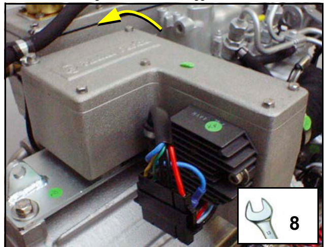
Fig. 9.8.0-1: Luftansauggehäuse
