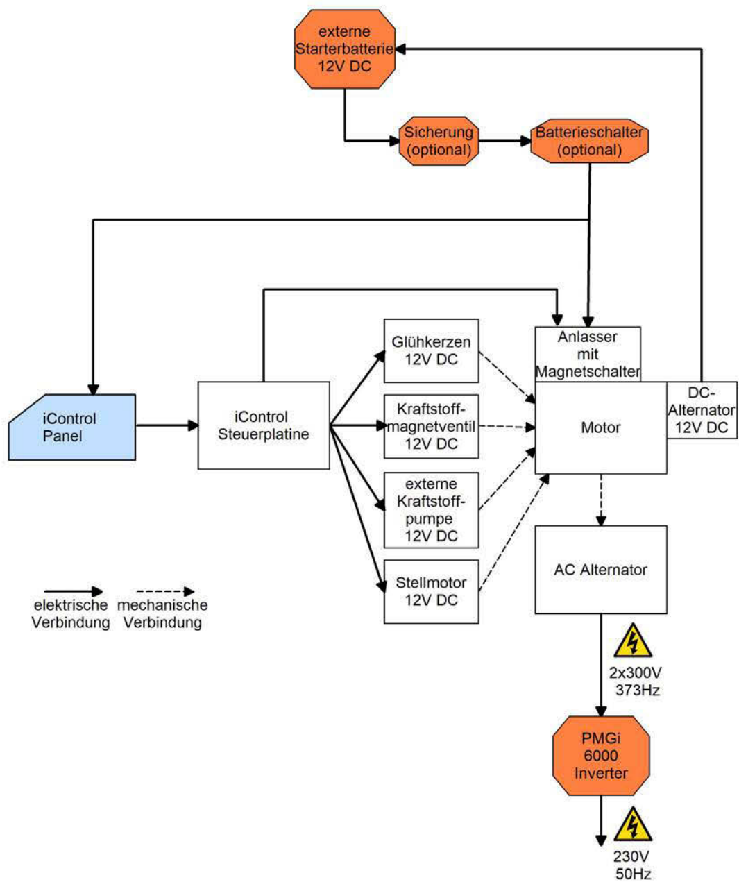
Fig. 6.3.4-1: Elektrisches System
