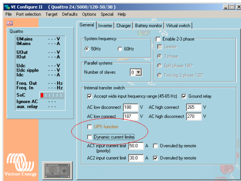
Fig. 19.7.1-1: Einstellungen in der Victron VE configure II Software
