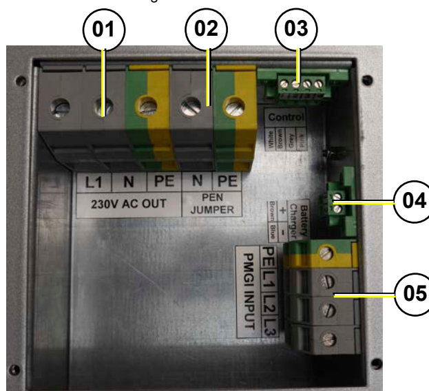
Fig. 12.4-1: Anschlussbox
