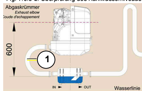
Fig. 7.6.3-2: Überprüfung des Kühlwasserniveaus
