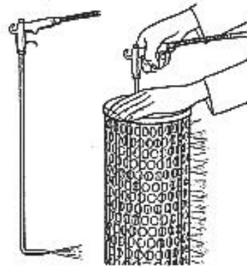
Fig. 9.9-8: Luftfilter reinigen
