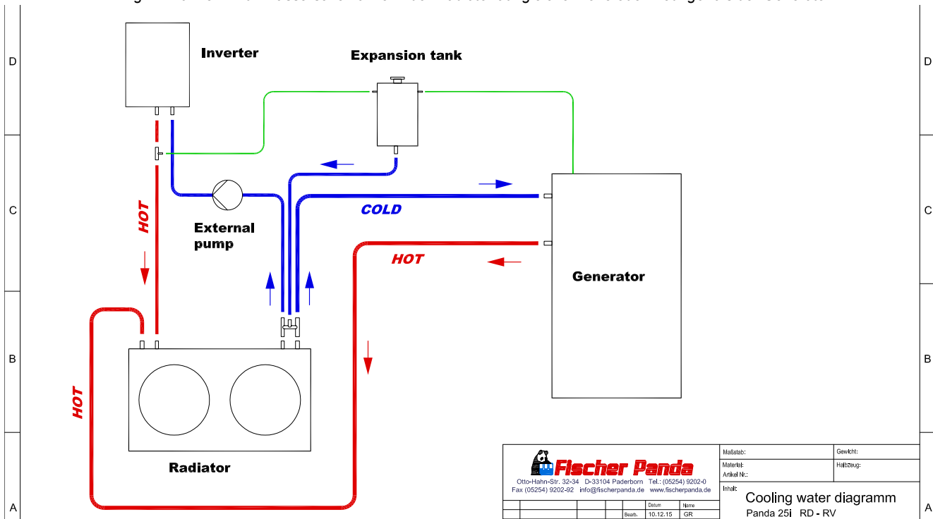
Fig. 12.10.1.3-2: Kühlwasserschema wenn der Radiator auf gleicher höhe oder niedriger als der Generator
