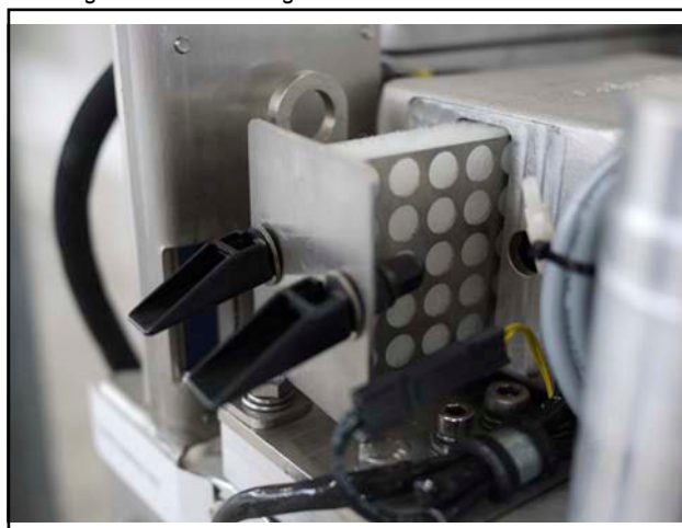
Fig. 9.8.1-3: Luftfiltergehäuse mit Schnellwechselhalter
