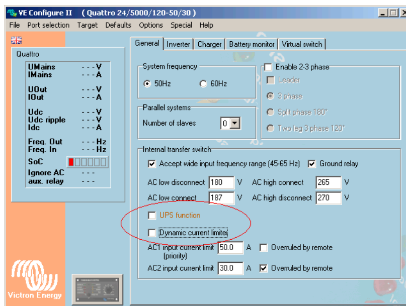
Fig. 12.6.1-1: Einstellungen in der Victron VE configure II Software
