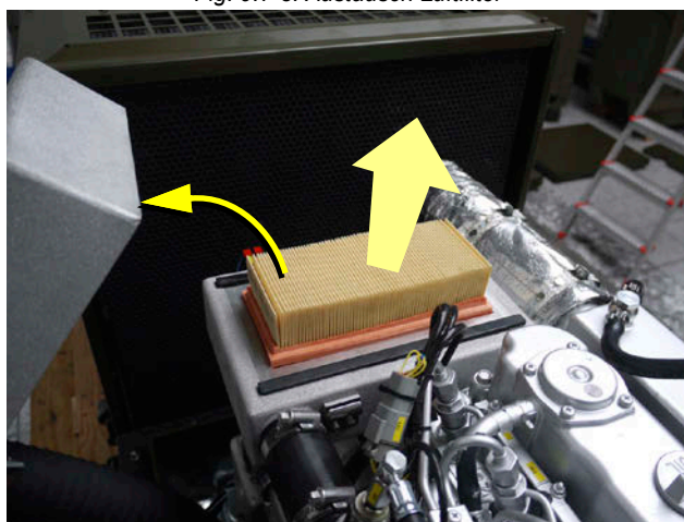
Fig. 9.7-3: Austausch Luftfilter
