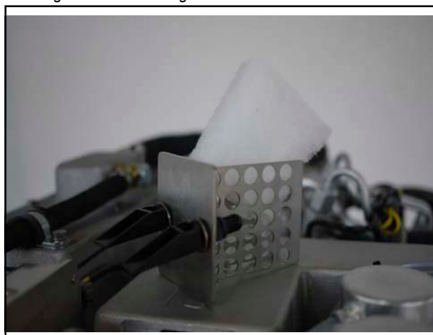
Fig. 9.8.1-4: Luftfiltergehäuse mit Schnellwechselhalter
