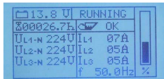
Fig. 15.3.3.4-3: Inverterseite Strangspannungen und Leiterströme
