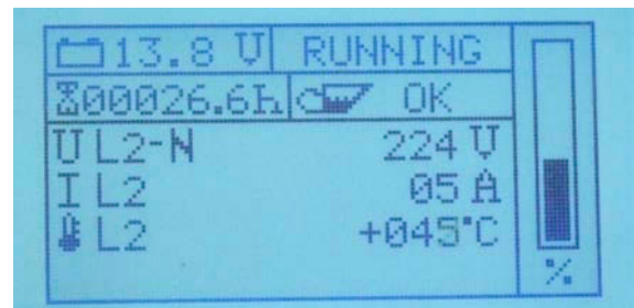
Fig. 15.3.3.4-6: Phasenspannung L2
