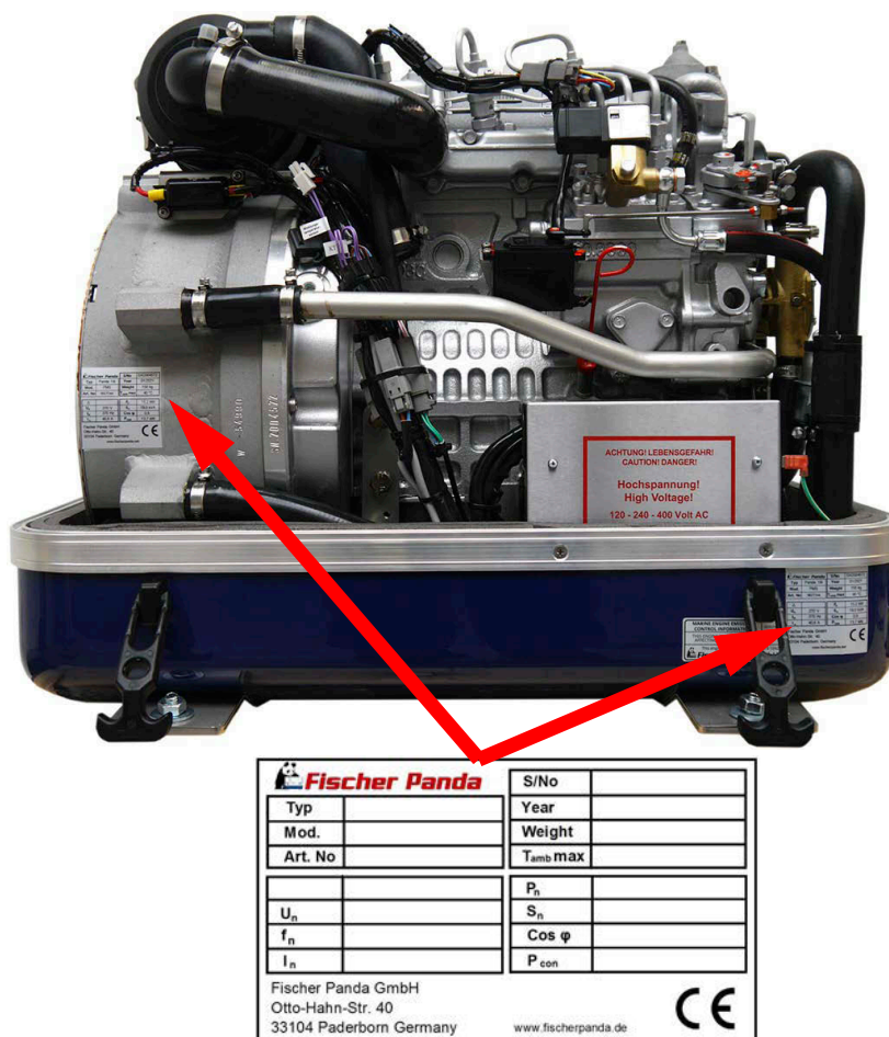
Fig. 6.1-2: Beschreibung des Typenschildes
