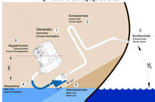
Fig. 7.6.3.1-3: Schräglage 30 Grad
