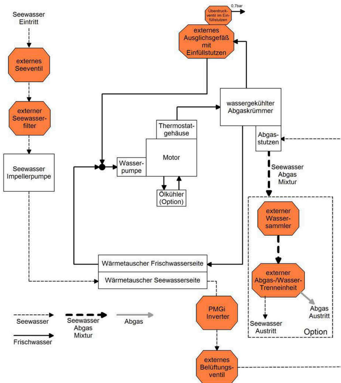
Fig. 6.4.1-1: Der Kühlkreislauf (See- und Frischwasser)
