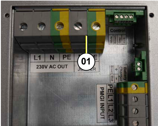
Fig. 12.10-1: PE-N Brücke
