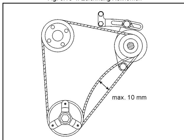
Fig. 9.15-4: Zeichnung Keilriemen
