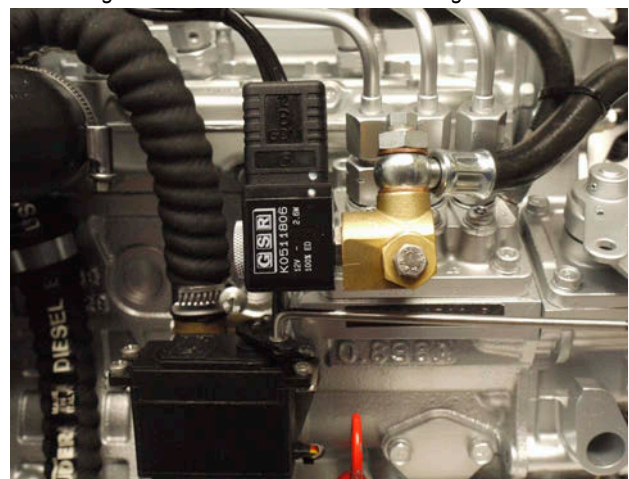
Fig. 10.4.1-1: Elektrisches Kraftstoffmagnetventil
