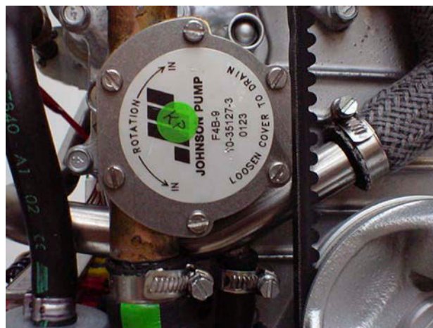
Fig. 9.5.3-3: Gehäuse Seewasserpumpe
