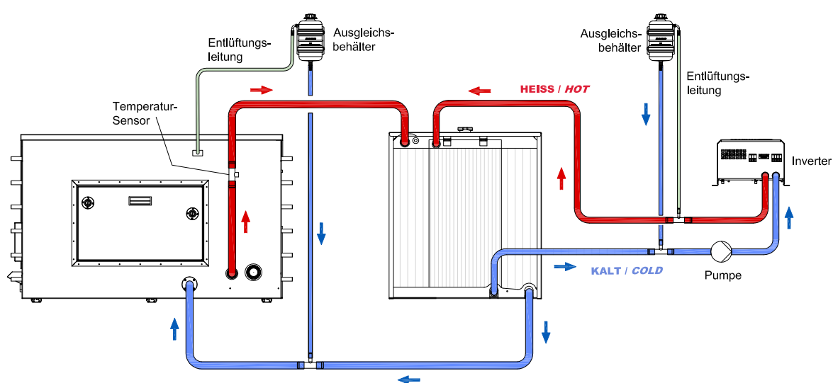
Fig. 12.10.1.3-1: Kühlwasserschema wenn der Radiator auf gleicher Höhe oder niedriger als der Generator
