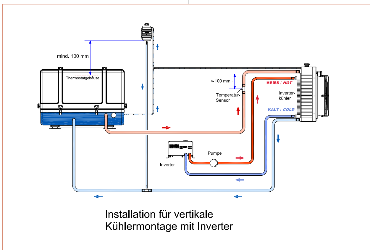
Fig. 12.10.1.2-1: Kühlwasserschema mit dem Radiator höher als der Generator
