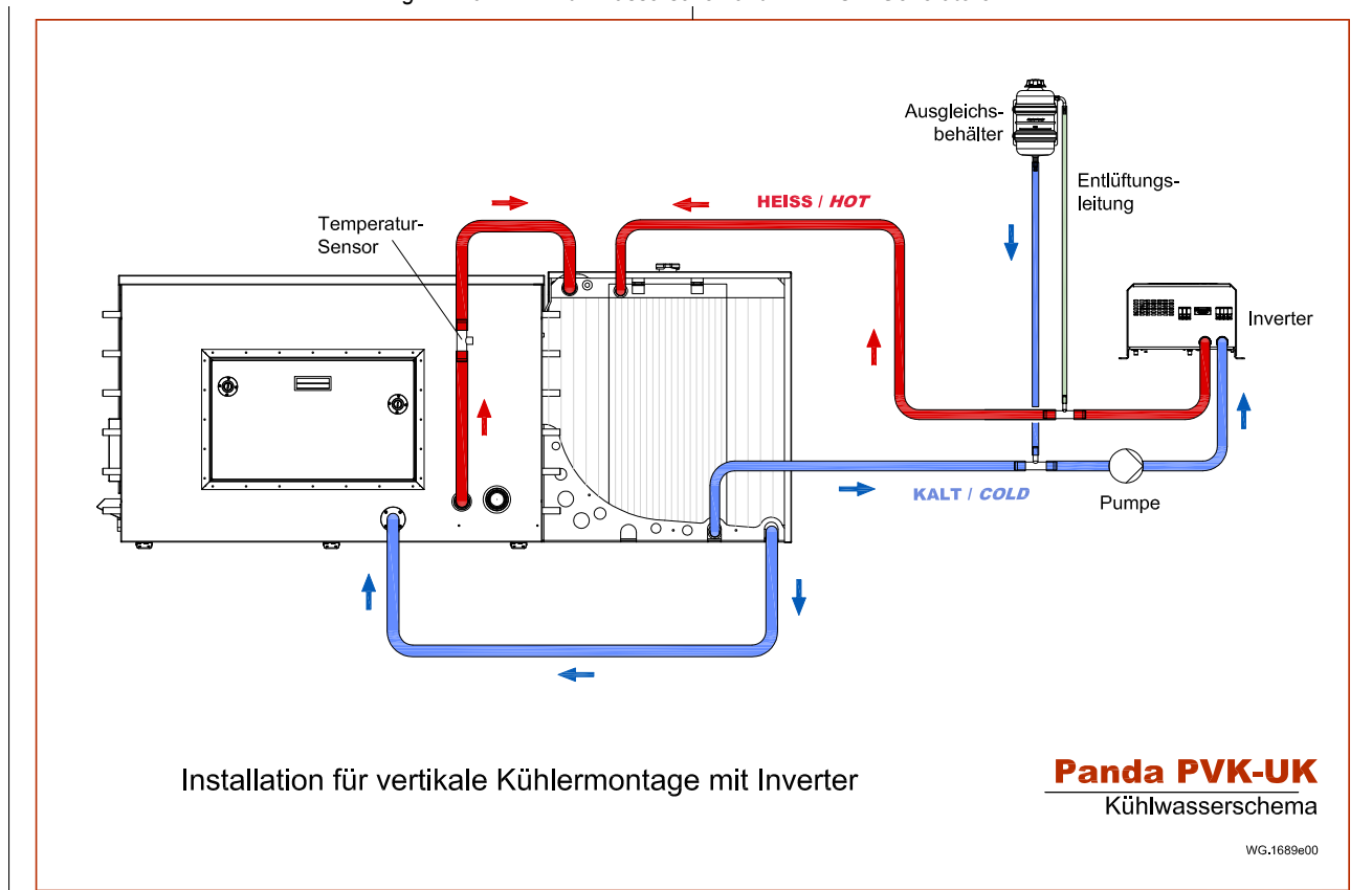
Fig. 12.10.1.4-1: Kühlwasserschema für PVK-UK iGeneratoren
