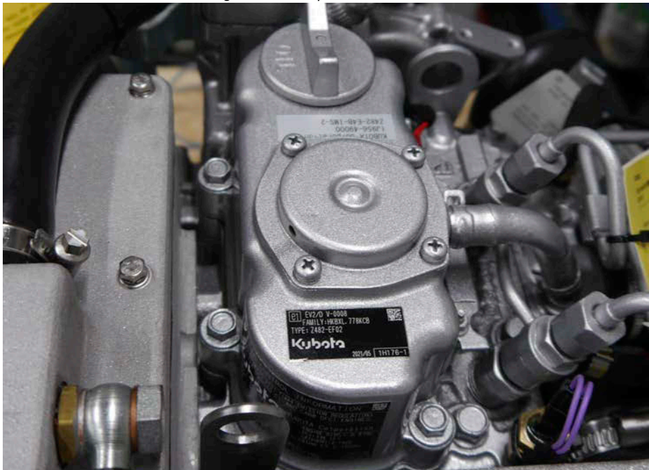
Fig. 19.4-2: Beispiel Z482 E4B IMS2
