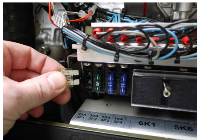
Fig. 9.14-3: Sicherung
