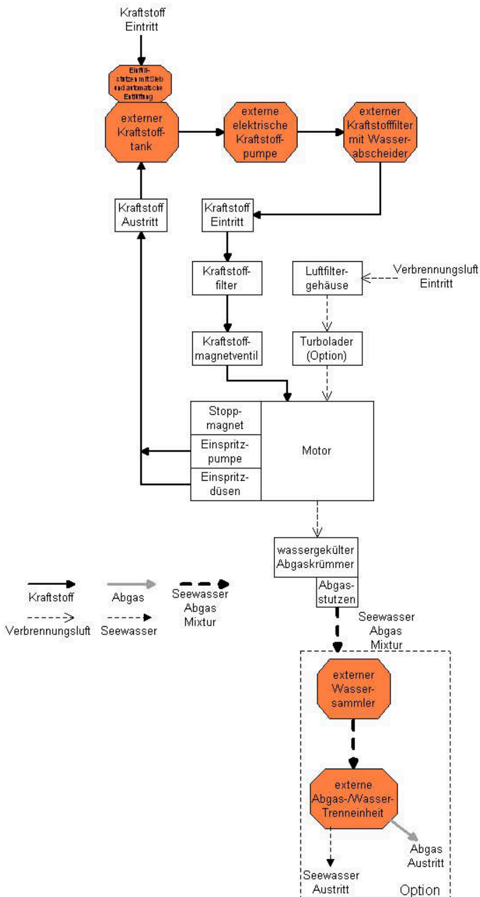
Fig. 6.4.2-1: Der Kraftstoff und Verbrennungsluft Kreislauf
