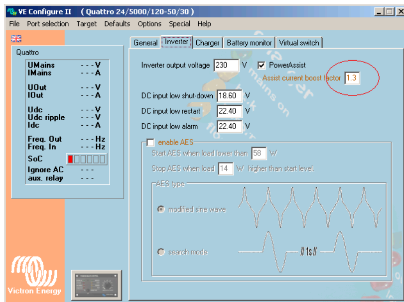
Fig. 12.6.2-1: Einstellungen in der Victron VE Configure II Software
