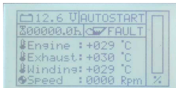
Fig. 15.3.3.7-1: Standard-Displayseite im Autostart-Modus
