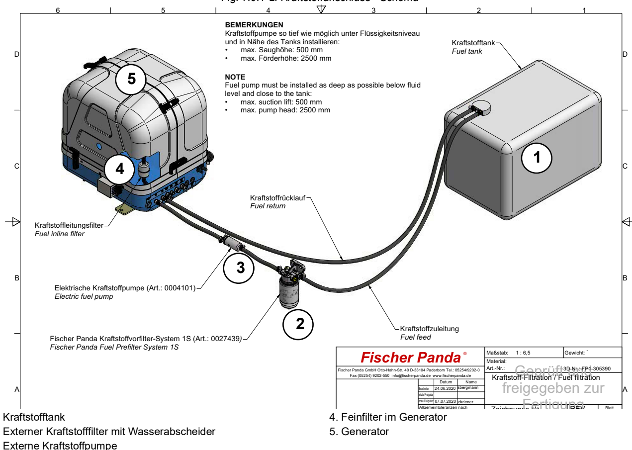
Fig. 7.9.1-2: Kraftstoffanschluss - Schema
