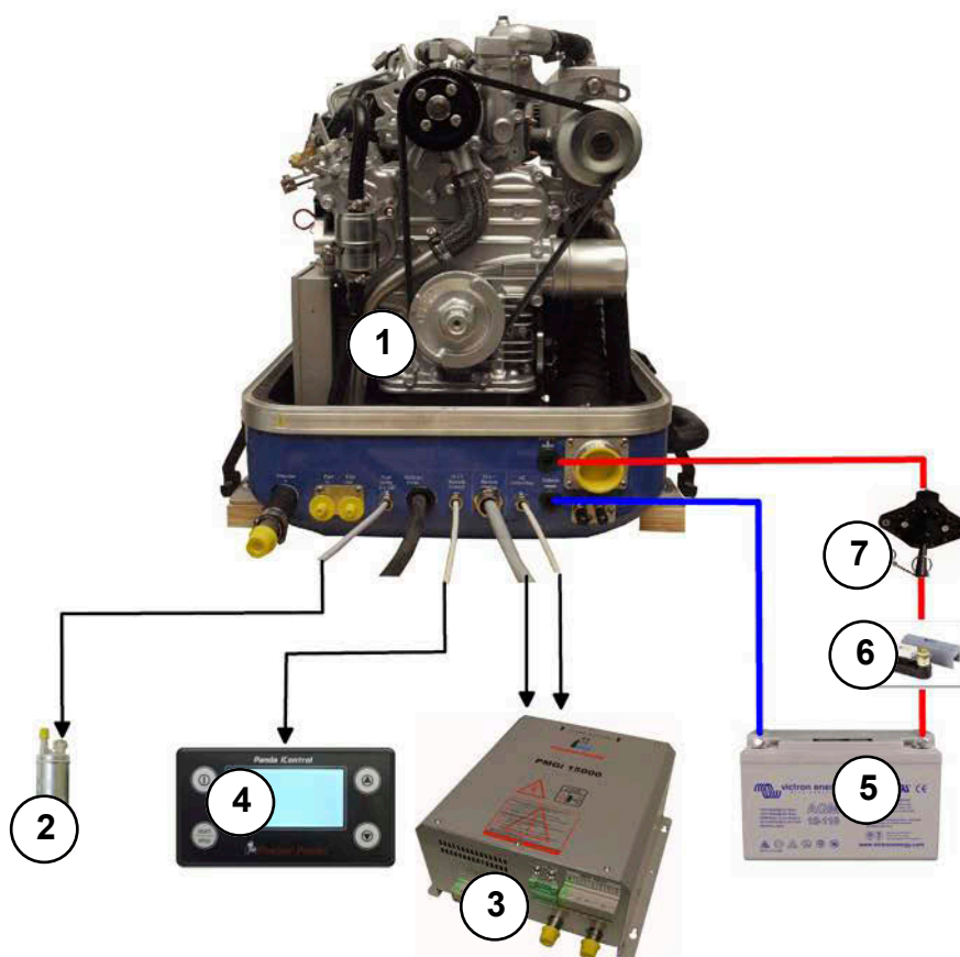
Fig. 7.11.0-1: Installationsschema Beispiel
