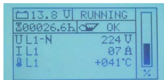
Fig. 15.3.3.4-5: Phasenspannung L1
