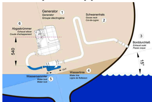
Fig. 7.6.3.1-2: Schräglage 15 Grad
