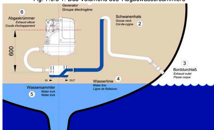
Fig. 7.6.3-1: Das Volumens des Abgaswassersammlers
