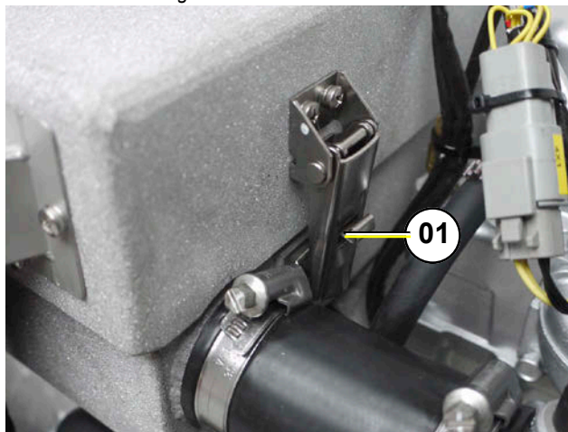
Fig. 9.7-2: Austausch Luftfilter
