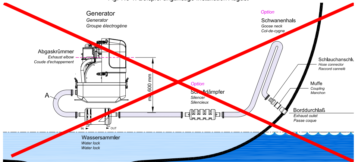
Fig. 7.8-1: Beispiel ungünstige Installation Abgast
