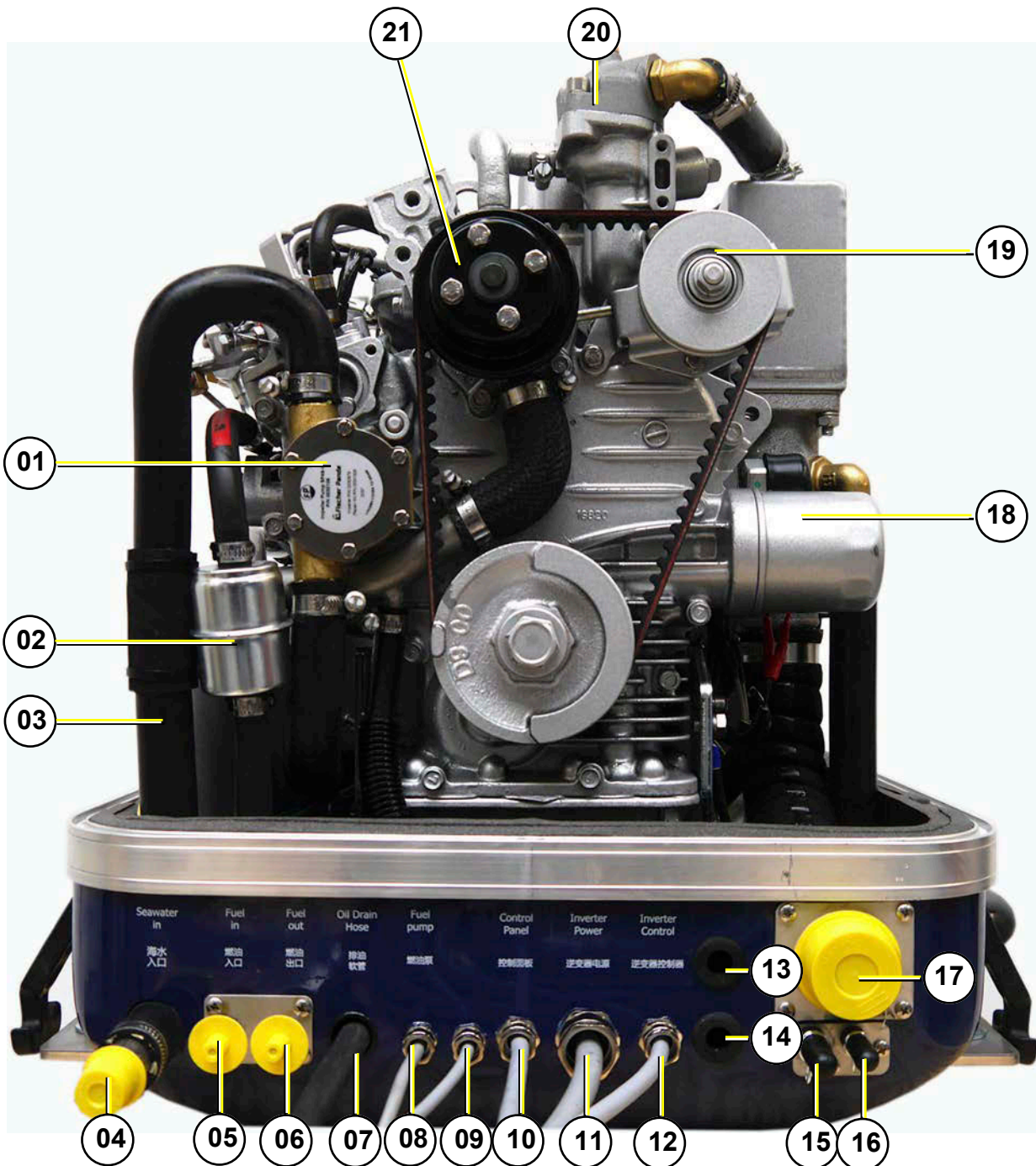
Fig. 6.2.3-1: Ansicht Vorderseite
