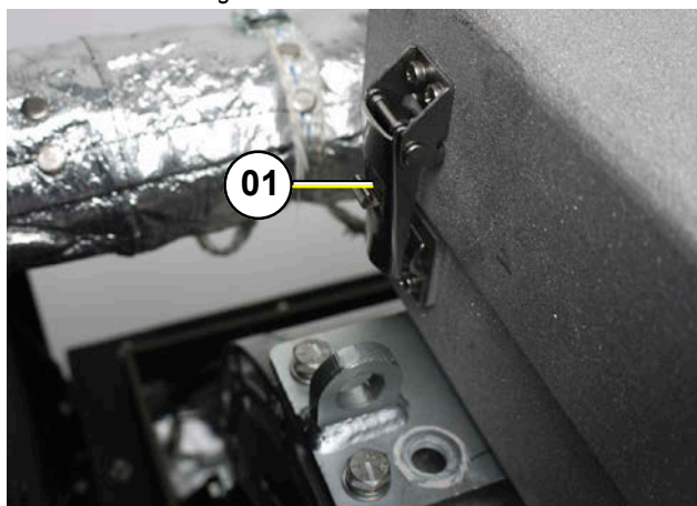
Fig. 9.7-3: Austausch Luftfilter
