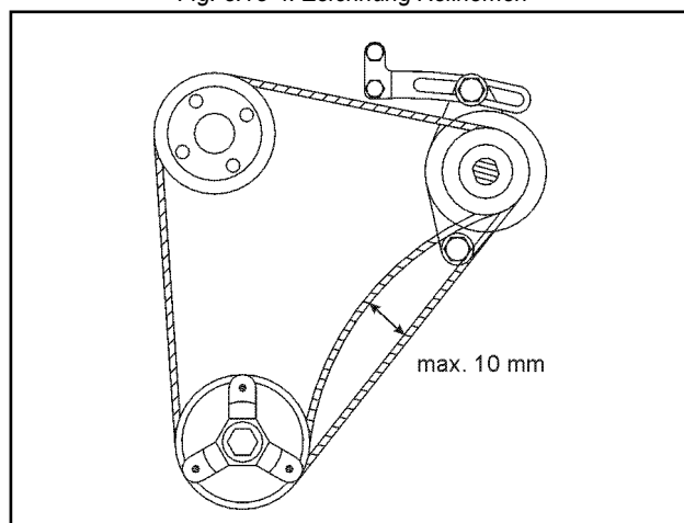
Fig. 8.15-4: Zeichnung Keilriemen
