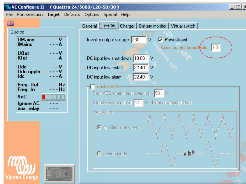
Fig. 11.7.2-1: Einstellungen in der Victron VE Configure II Software
