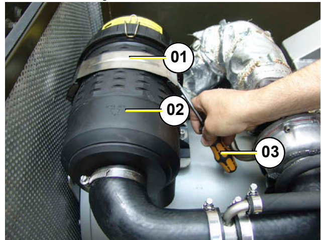
Fig. 8.9-1: Austausch Luftfilter
