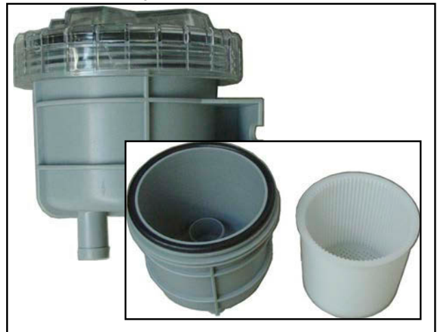
Fig. 8.5.1-1: Seewasserfilter
