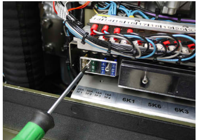
Fig. 8.14-2: Sicherung
