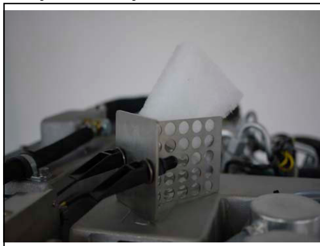
Fig. 8.8.1-4: Luftfiltergehäuse mit Schnellwechselhalter
