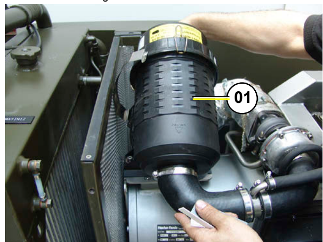
Fig. 8.9-2: Austausch Luftfilter
