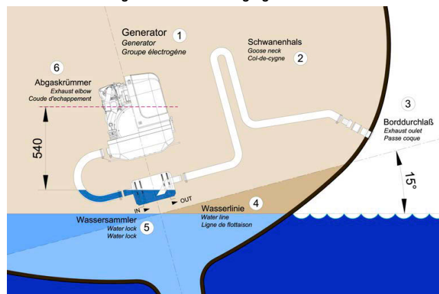
Fig. 6.6.3.1-2: Schräglage 15 Grad
