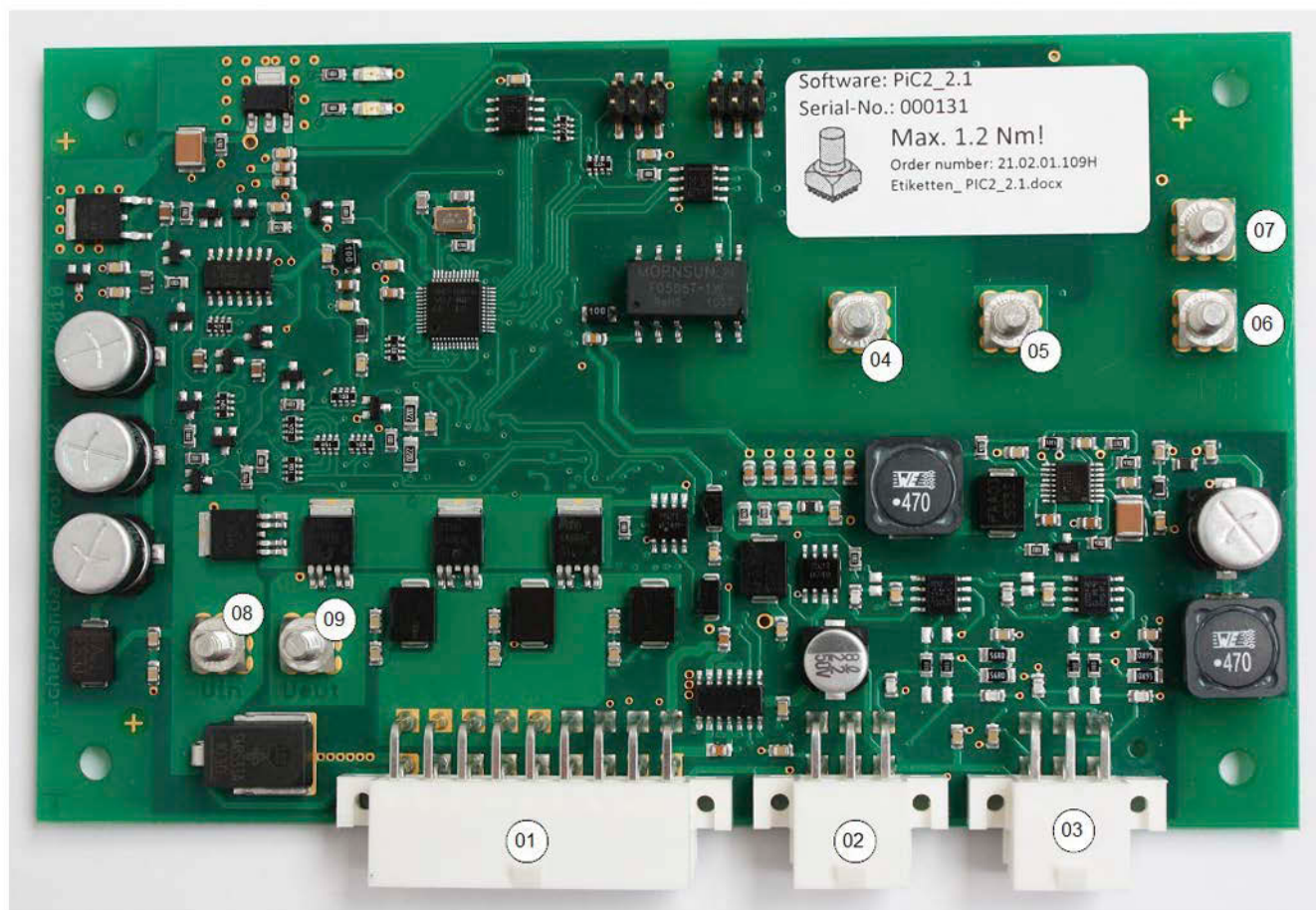
Fig. 15.4-1: Beschaltung des Panda iControl2-Steuergerätes
