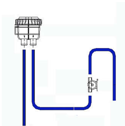
Fig. 6.4.4-1: Schleife in der Kühlwasserleitung vor dem Impeller
