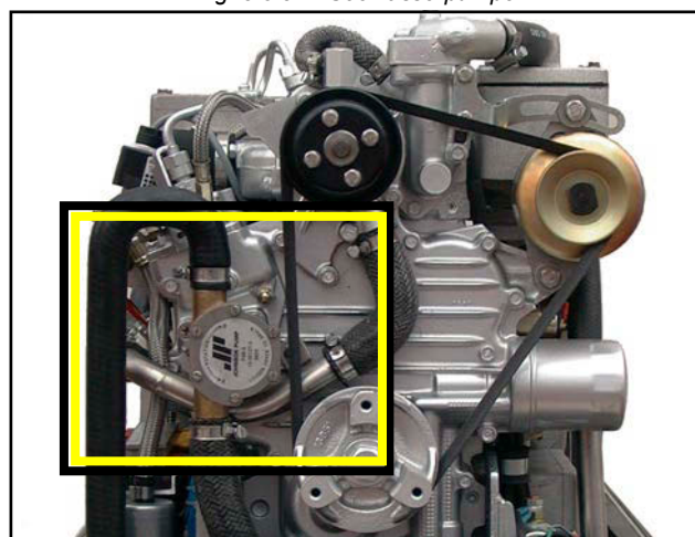
Fig. 8.5.3-3: Gehäuse Seewasserpumpe
