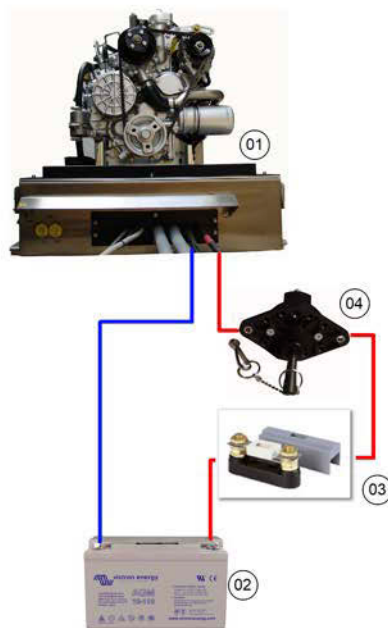
Fig. 6.10.3-1: Starterbatterieanschluss 12 V- Schema
