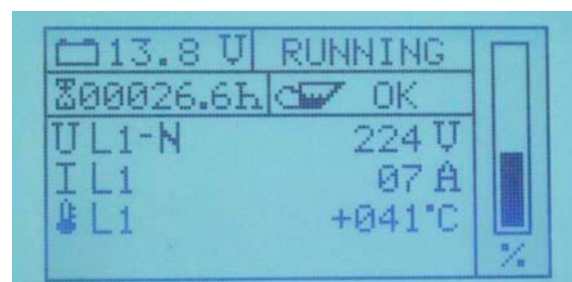
Fig. 14.3.3.4-5: Phasenspannung L1
