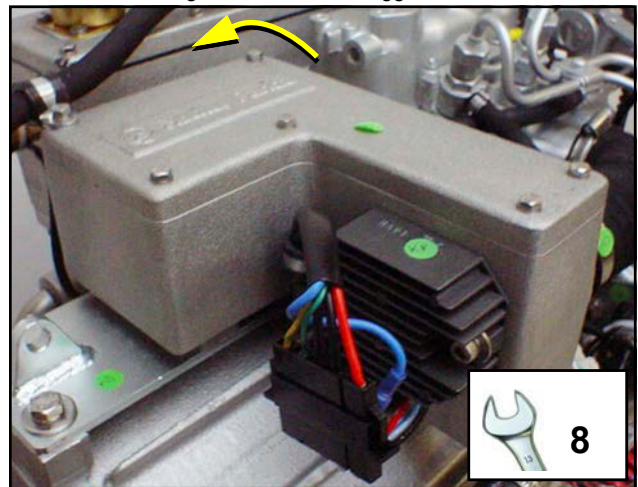
Fig. 8.8.0-1: Luftansauggehäuse
