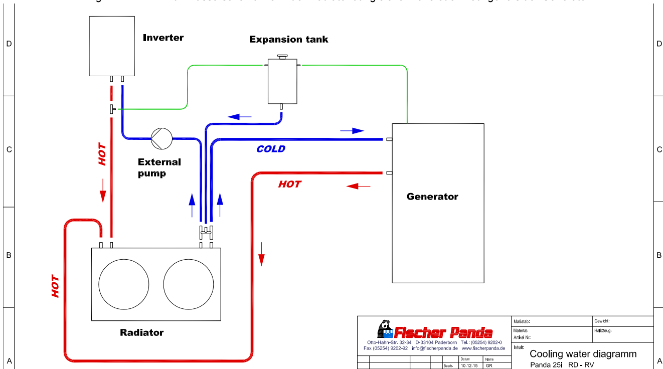
Fig. 11.11.1.1-1: Kühlwasserschema wenn der Radiator auf gleicher höhe oder niedriger als der Generator
