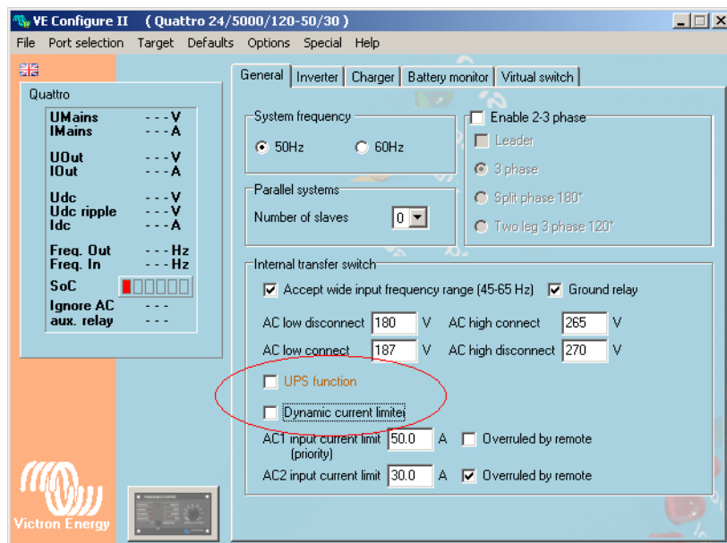
Fig. 11.7.1-1: Einstellungen in der Victron VE configure II Software
