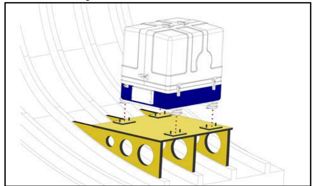
Fig. 6.2.3-1: Generator-Fundament
