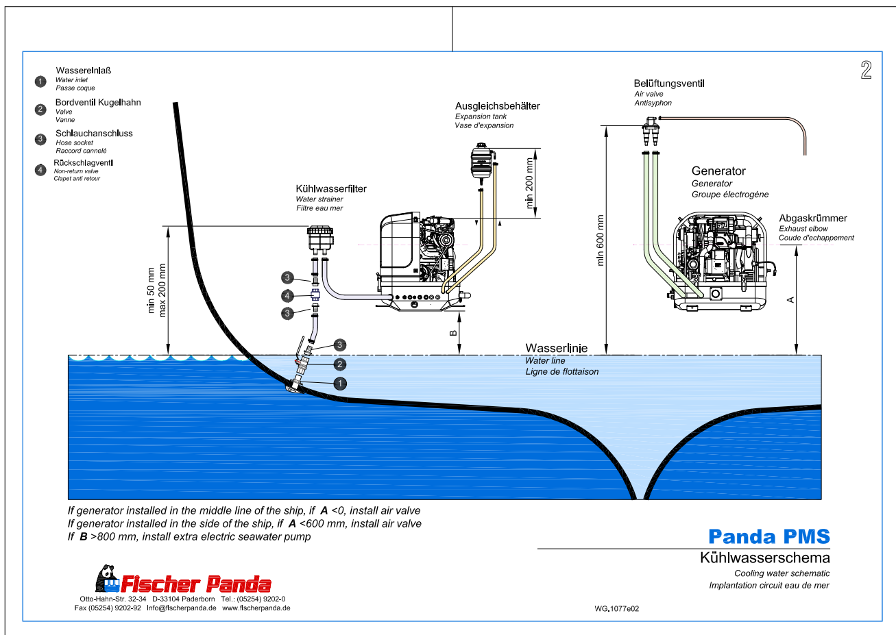
Fig. 6.4.4.1-1: Installationsschema Seewasserkühlung über Wärmetauscher
