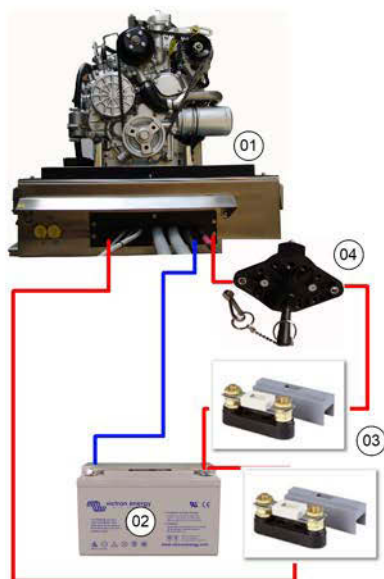
Fig. 6.10.3-3: Starterbatterieanschluss 12 V- Schema mit seperatem Stromanschluss für die ECU
