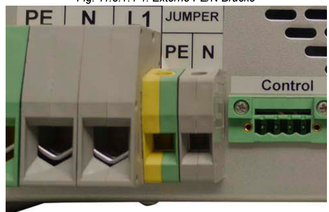
Fig. 11.5.1.4-1: Externe PE/N Brücke
