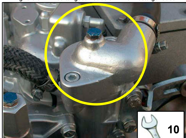
Fig. 8.6.3-2: Entlüftungsschraube am Thermostatgehäuse
