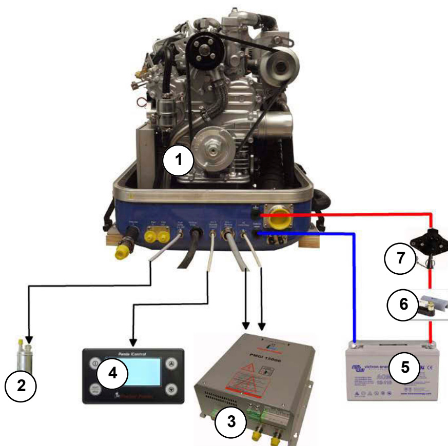
Fig. 6.11.0-1: Installationsschema Beispiel
