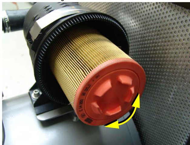
Fig. 8.9-4: Austausch Luftfilter
