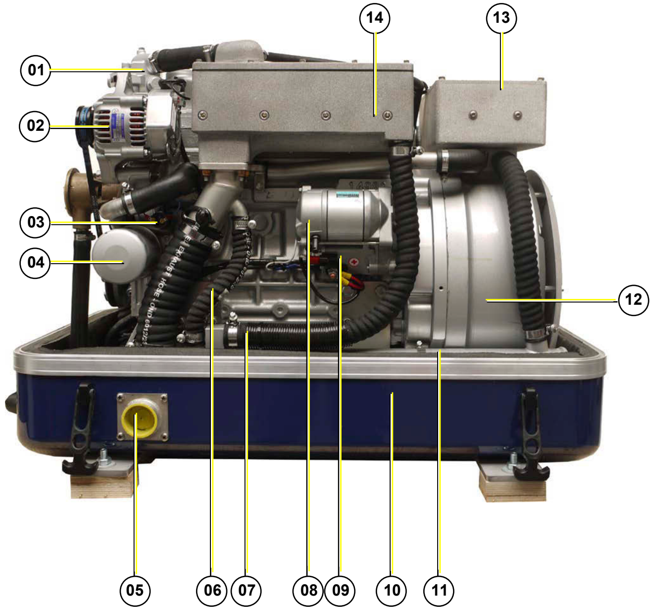
Fig. 5.2.1-1: Seitenansicht Rechts
