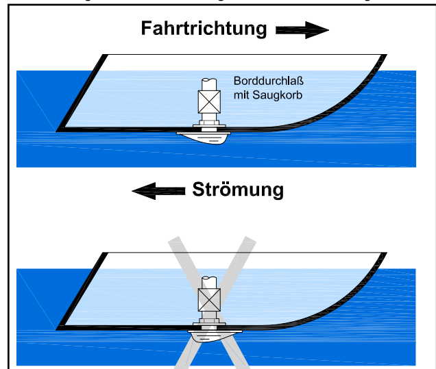
Fig. 6.4.2-1: Anordnung der Borddurchführung
