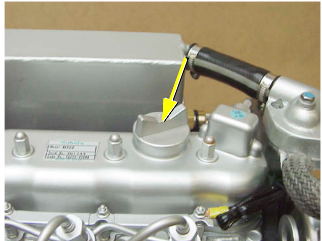
Fig. 8.11-1: Öleinfülldeckel
