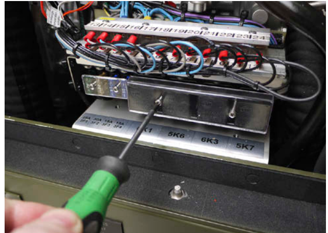
Fig. 8.13-1: Relais
