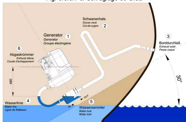
Fig. 6.6.3.1-3: Schräglage 30 Grad
