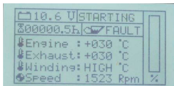
Fig. 17.1.1-2: Warnung „Wicklung“ zu hoch
