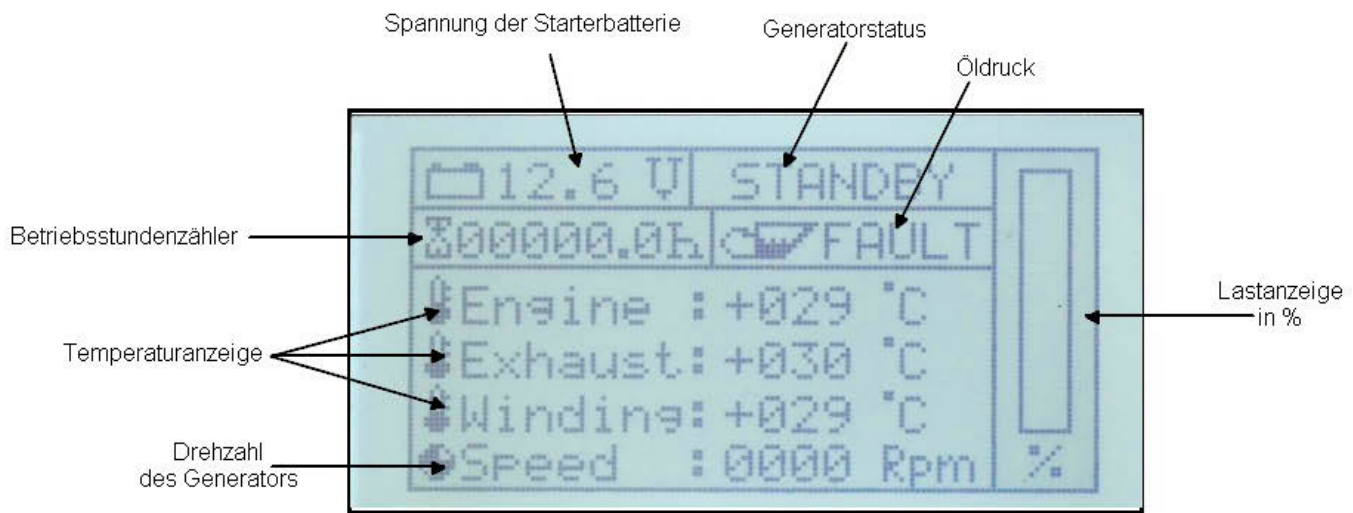
Fig. 14.3.2-1: Standard Displayseite
