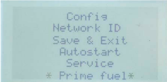
Fig. 14.4.1-2: Setup-Menü
