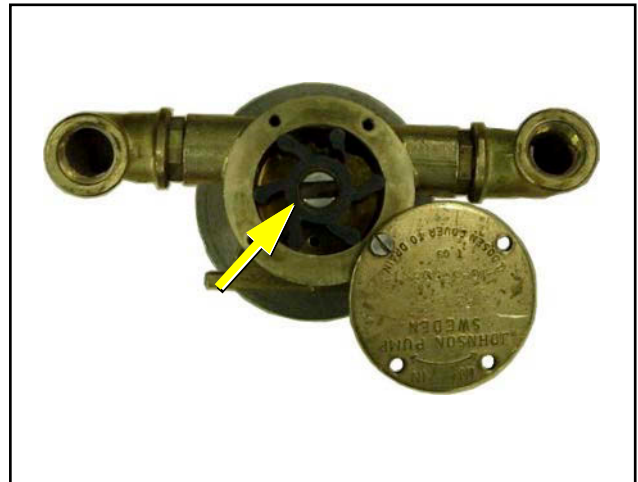
Fig. 8.5.3-4: Impeller
