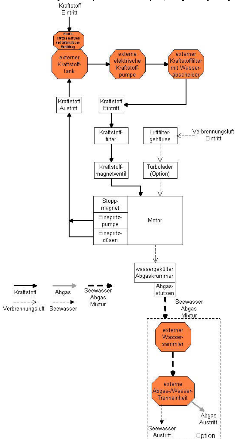
Fig. 5.4.2-1: Komponenten des Kraftstoffsystem, Ansaugluftführung und Abgassystems
