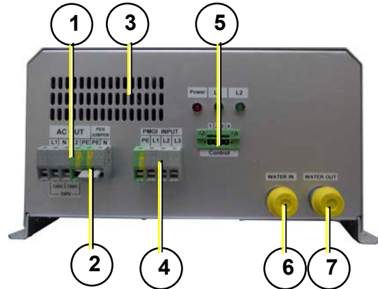
Fig. 11.5-1: Anschlussseite
