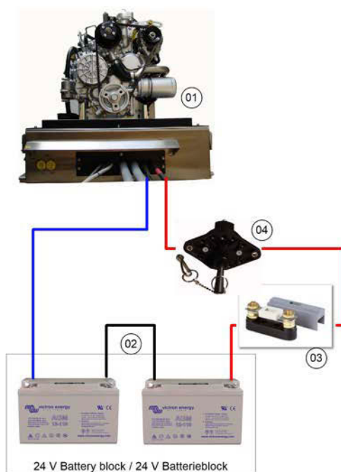
Fig. 6.10.3-2: Starterbatterieanschluss 24 V - Schema
