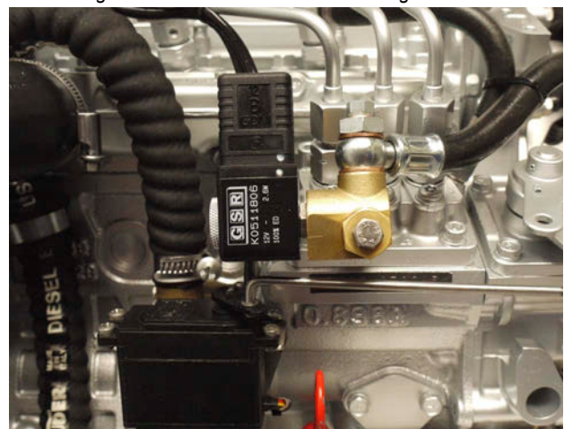
Fig. 9.4.1-1: Elektrisches Kraftstoffmagnetventil
