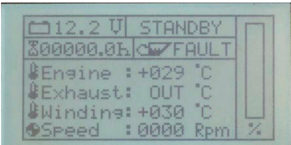
Fig. 17.2.0-1: Fehler „Zylinderkopftemperatur out of range“
