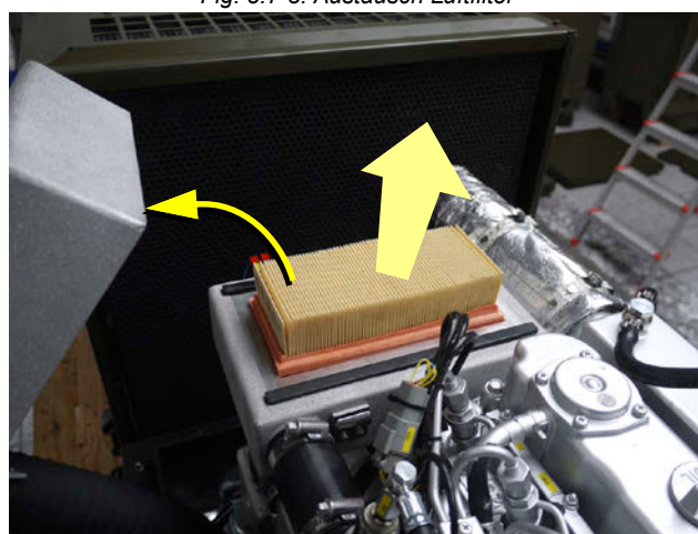
Fig. 8.7-3: Austausch Luftfilter
