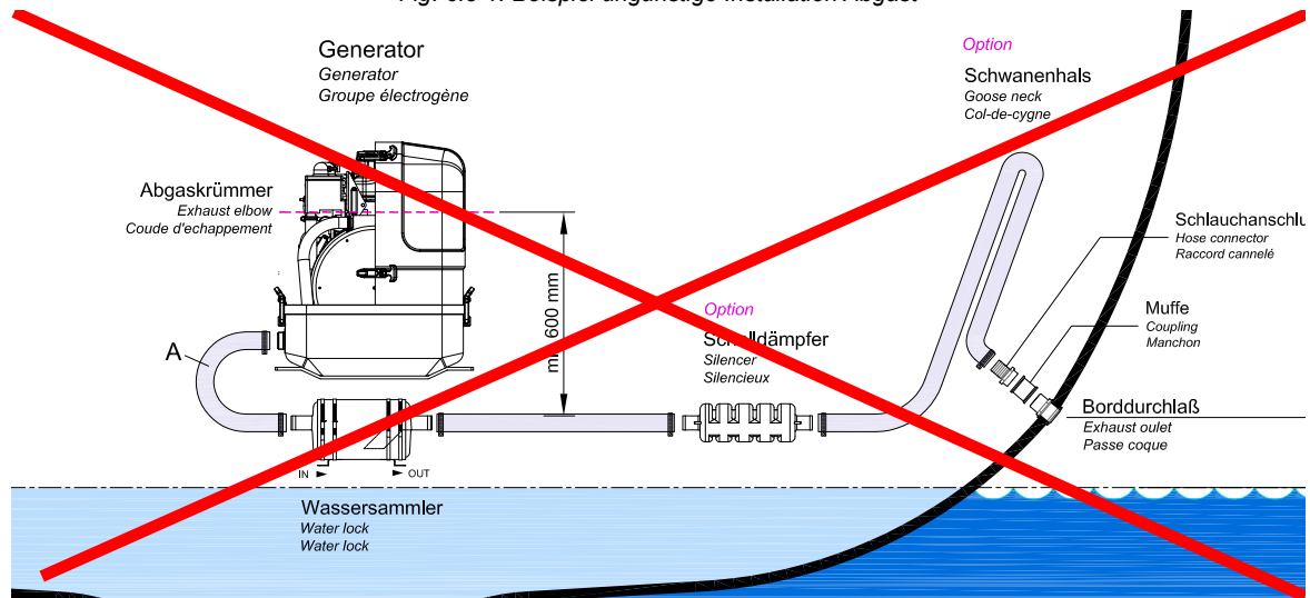
Fig. 6.8-1: Beispiel ungünstige Installation Abgast
