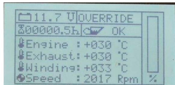
Fig. 14.3.3.3-1: Standard-Displayseite während des Override-Modus
