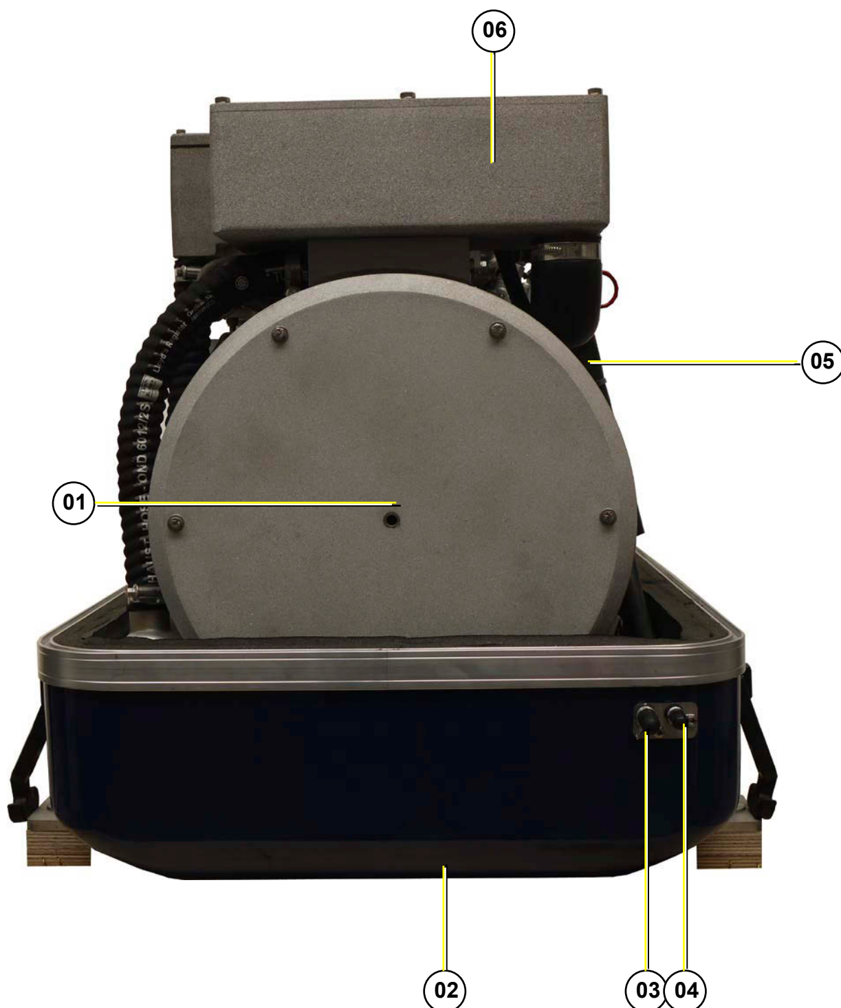
Fig. 5.2.4-1: Rückseite
