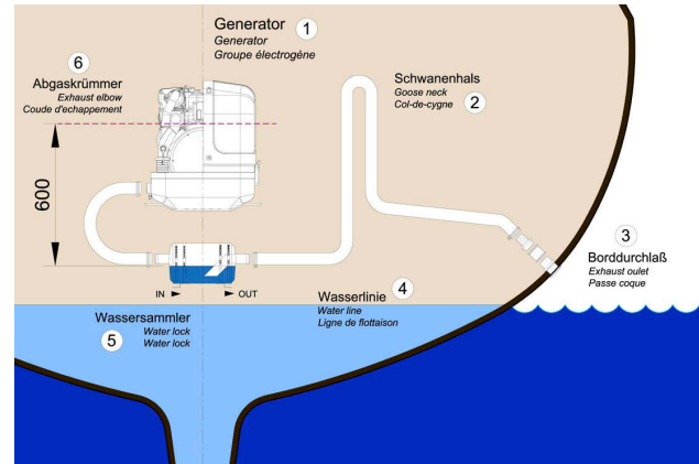
Fig. 6.6.3.1-1: Idealposition des Wassersammlers
