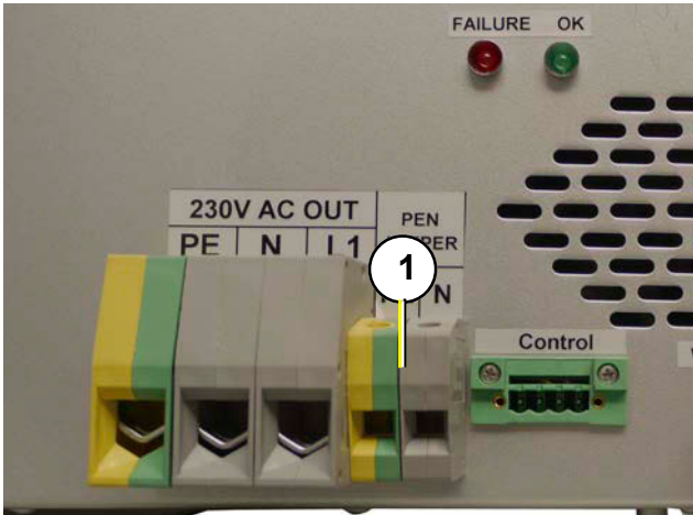
Fig. 11.11-1: PE-N Brücke
