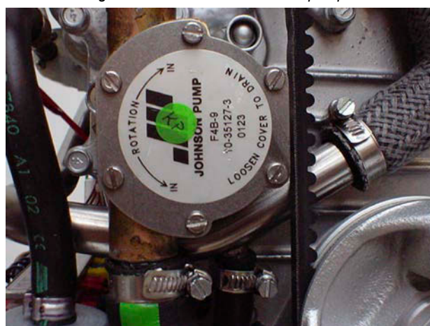
Fig. 8.5.3-3: Gehäuse Seewasserpumpe
