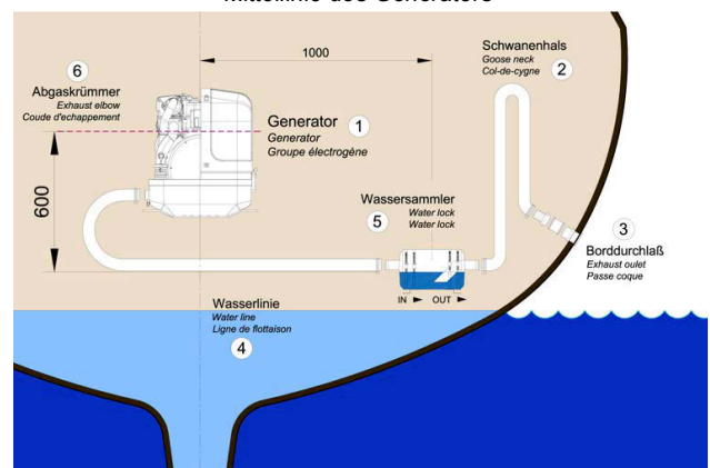
Fig. 6.6.3.2-3: Abgaswassersammler 1000 mm neben der Mittellinie des Generators
