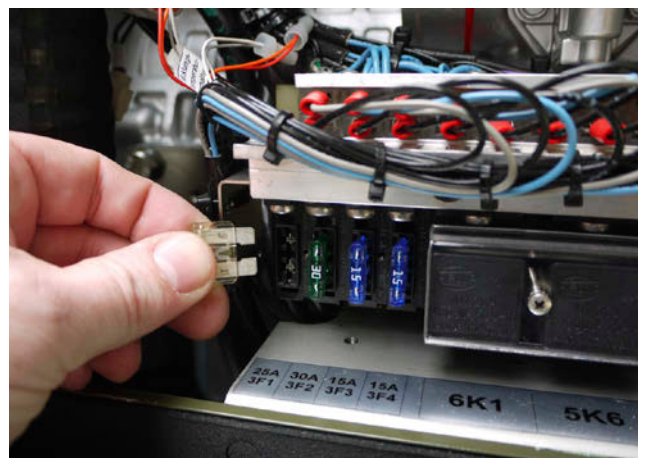
Fig. 8.14-3: Sicherung
