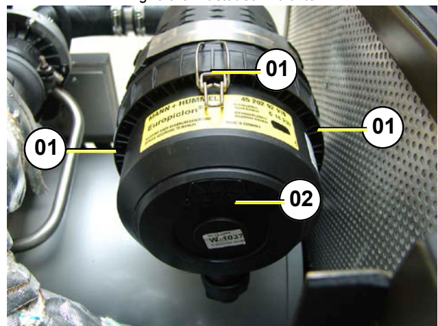
Fig. 8.9-3: Austausch Luftfilter
