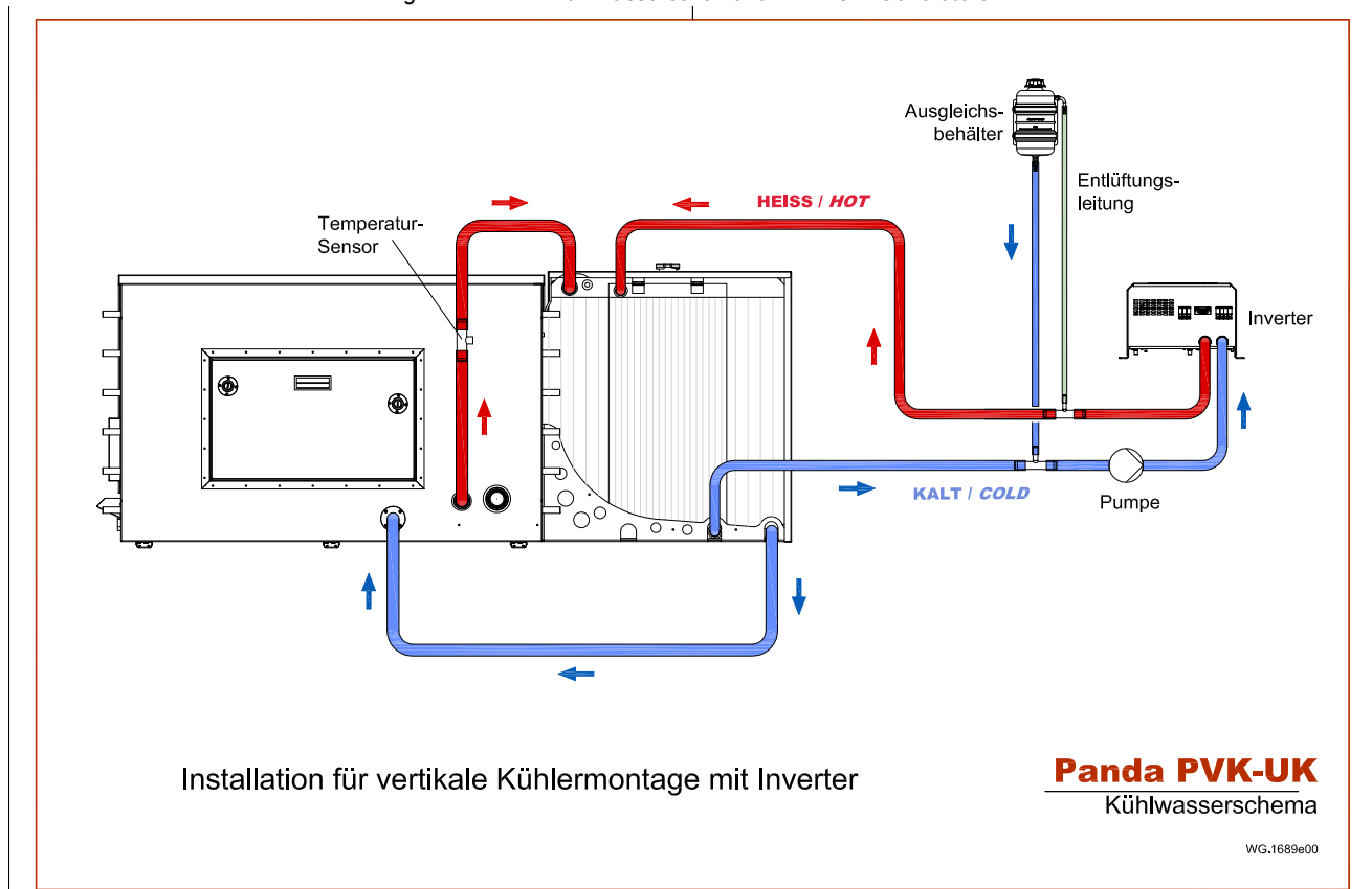
Fig. 11.11.1.2-1: Kühlwasserschema für PVK-UK iGeneratoren
