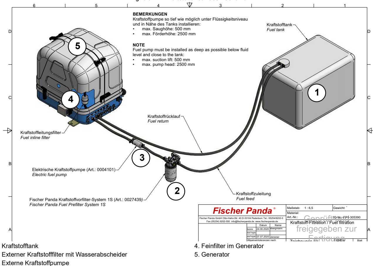
Fig. 6.9.1-2: Kraftstoffanschluss - Schema
