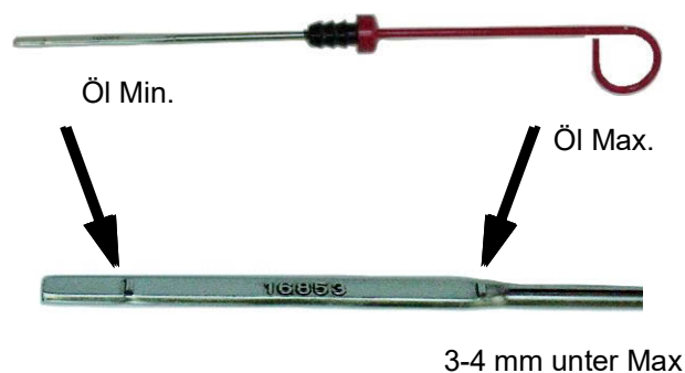
Fig. 8.10.1-1: Ölpeilstab - Beispiel
