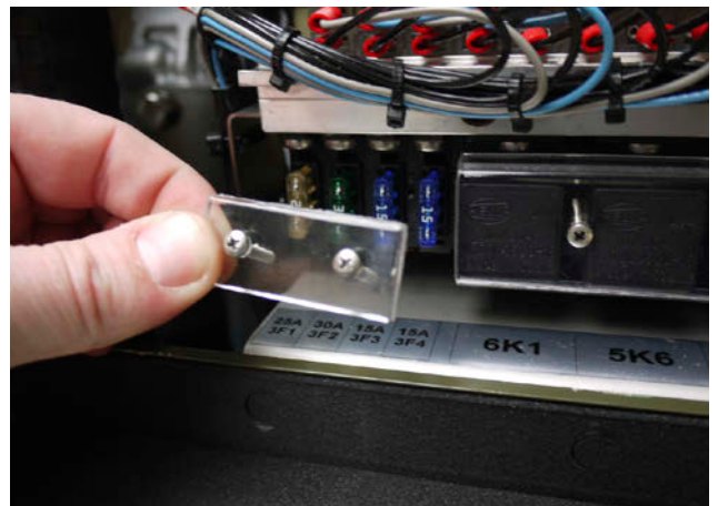
Fig. 8.14-2: Sicherung
