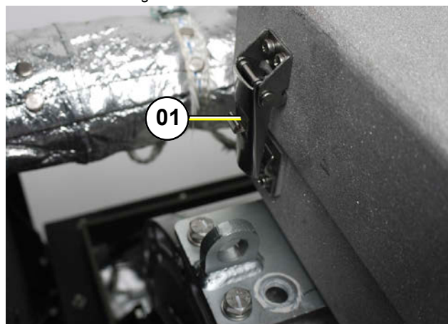
Fig. 8.7-3: Austausch Luftfilter
