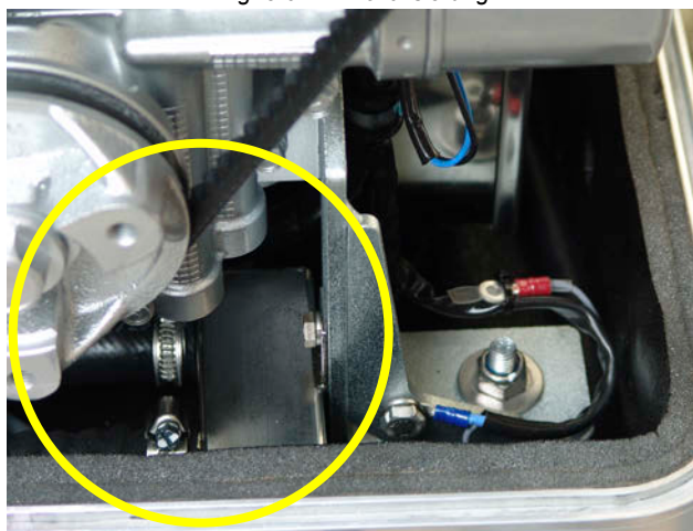
Fig. 8.6.2-1: Lokalisierung
