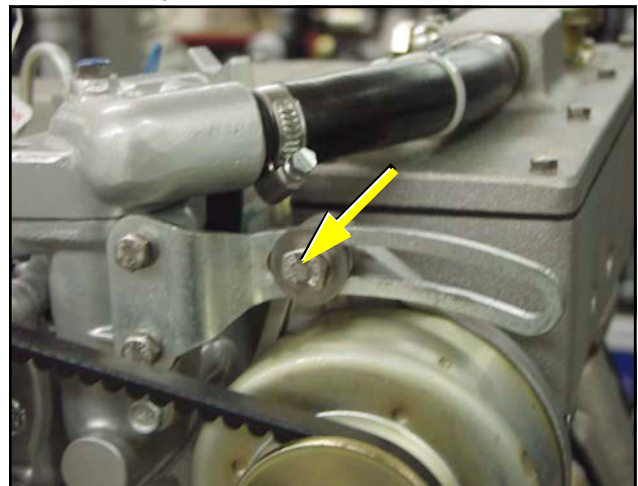
Fig. 8.15-1: Lichtmaschinen-Schraube
