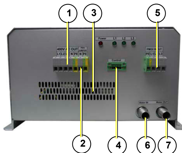
Fig. 11.4-1: Anschlussseite
