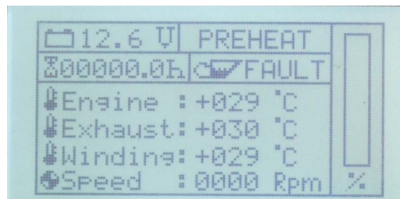
Fig. 15.3.3.2-1: Standard-Displayseite während des Vorglühens
