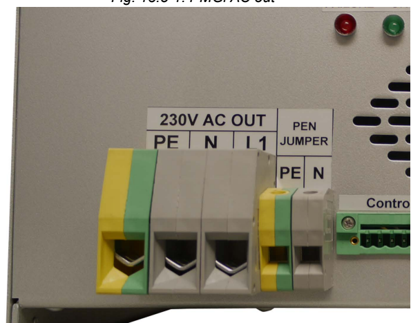
Fig. 13.5-1: PMGi AC out
