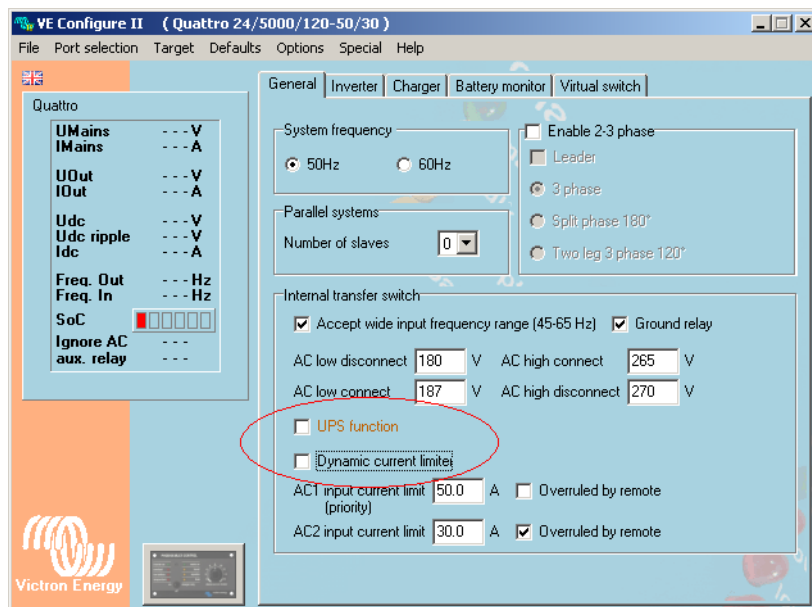
Fig. 13.7.1-1: Einstellungen in der Victron VE configure II Software
