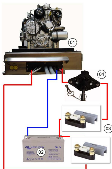
Fig. 8.10.3-3: Starterbatterieanschluss 12 V- Schema mit seperatem Stromanschluss für die ECU
