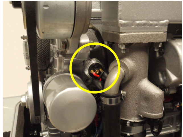
Fig. 7.3.6-4: Öldruckschalter
