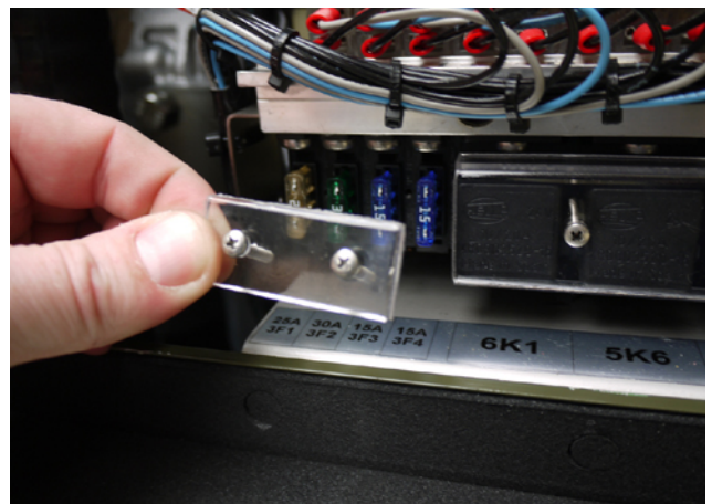
Fig. 10.14-2: Sicherung
