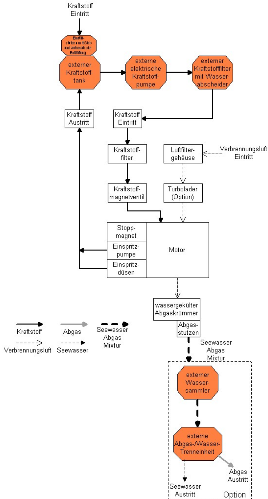
Fig. 7.3.3-1: Kraftstoffsystem, Ansaugluftführung und Abgassystem
