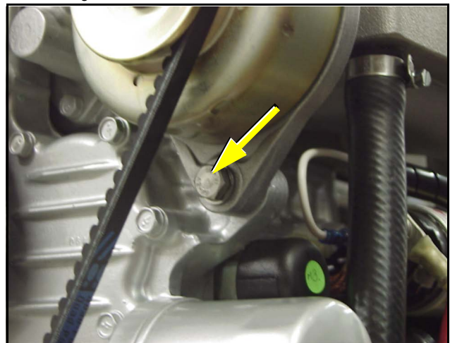
Fig. 10.15-2: Schraube unter der Lichtmaschine
