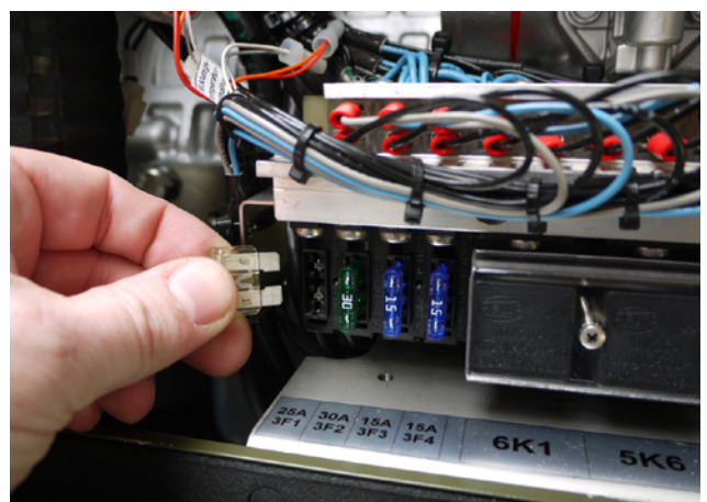
Fig. 10.14-3: Sicherung
