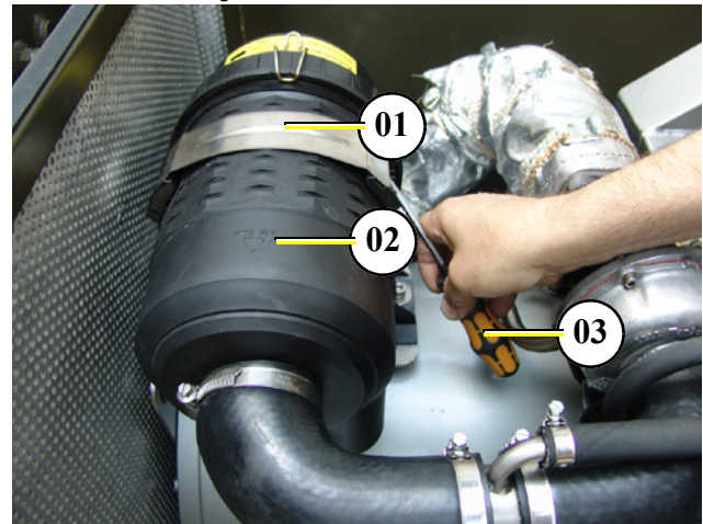
Fig. 10.9-1: Austausch Luftfilter
