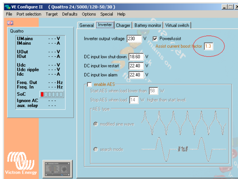
Fig. 13.7.2-1: Einstellungen in der Victron VE Configure II Software
