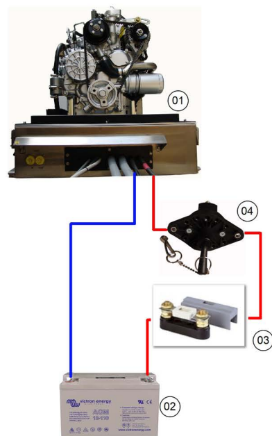
Fig. 8.10.3-1: Starterbatterieanschluss 12 V- Schema
