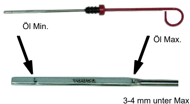
Fig. 10.10.1-1: Ölpeilstab - Beispiel
