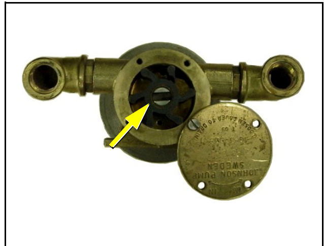
Fig. 10.5.3-4: Impeller
