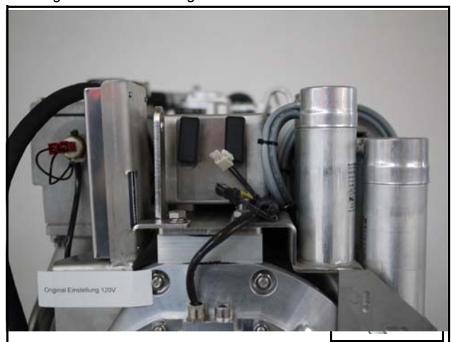
Fig. 10.8.1-1: Luftfiltergehäuse mit Schnellwechselhalter
