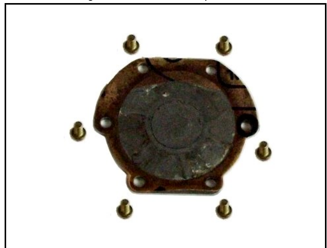
Fig. 10.5.3-6: Deckel Pumpenwelle
