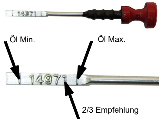
Fig. 10.10.1-2: Beispielbild Ölpeilstab
