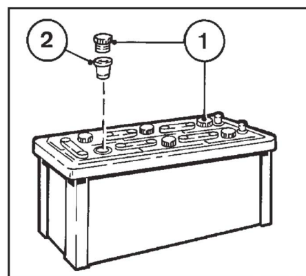
Fig. 10.12.1.2-1: Batterie
