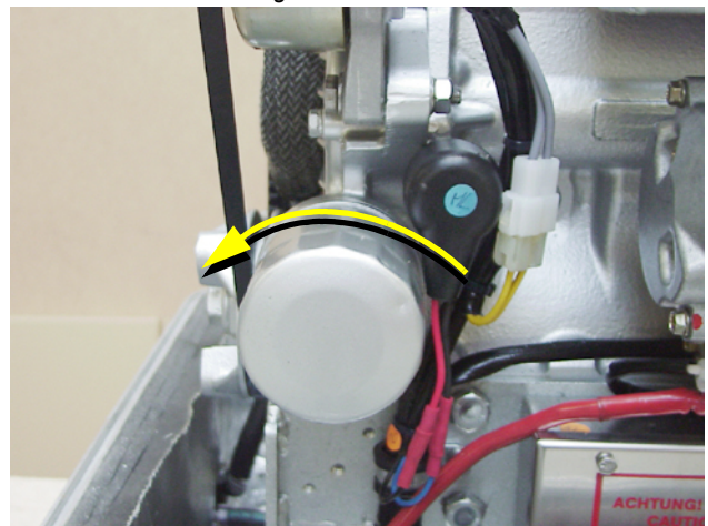
Fig. 10.11-3: Ölfilter
