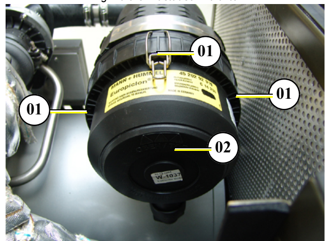
Fig. 10.9-3: Austausch Luftfilter
