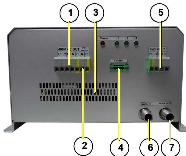
Fig. 13.4-1: Anschlussseite
