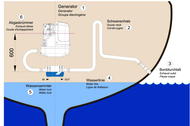
Fig. 8.6.3.1-1: Idealposition des Wassersammlers
