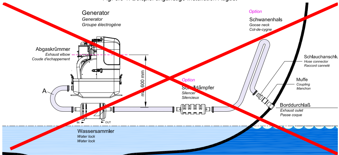
Fig. 8.8-1: Beispiel ungünstige Installation Abgast
