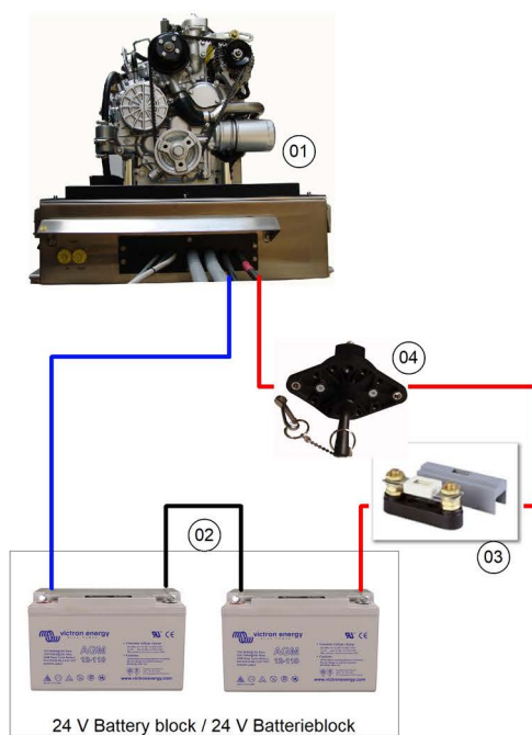
Fig. 8.10.3-2: Starterbatterieanschluss 24 V - Schema
