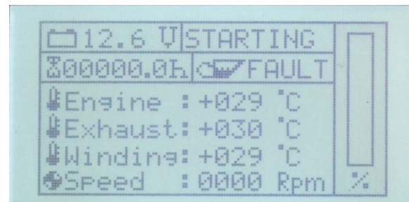
Fig. 15.3.3.2-2: Standard-Displayseite während des Startens
