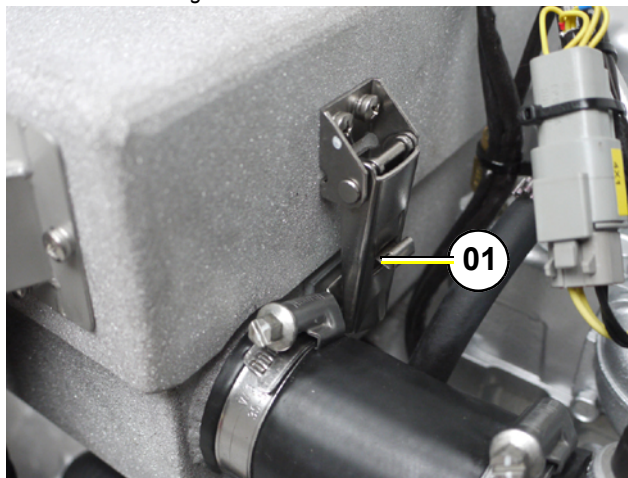
Fig. 10.7-2: Austausch Luftfilter
