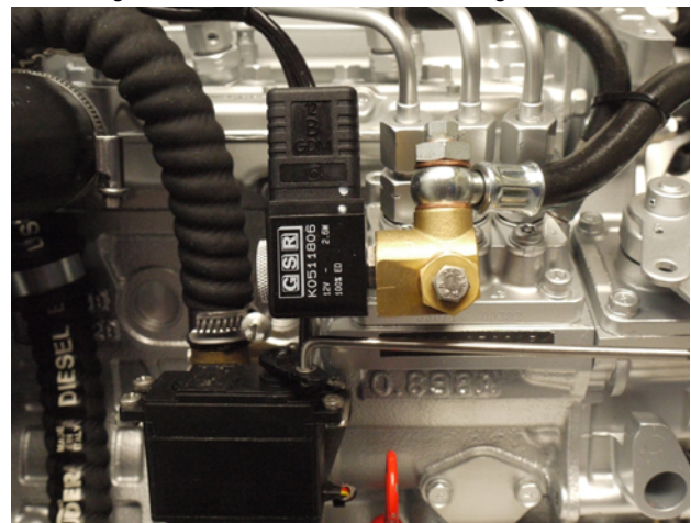
Fig. 11.4.1-1: Elektrisches Kraftstoffmagnetventil
