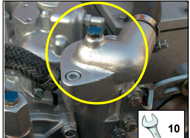
Fig. 10.6.3-2: Entlüftungsschraube am Thermostatgehäuse
