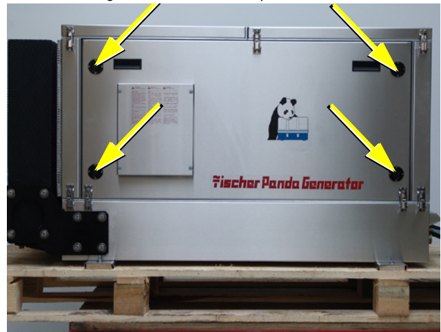
Fig. 5.5-1: Schalldämmkapsel Seitenteil
