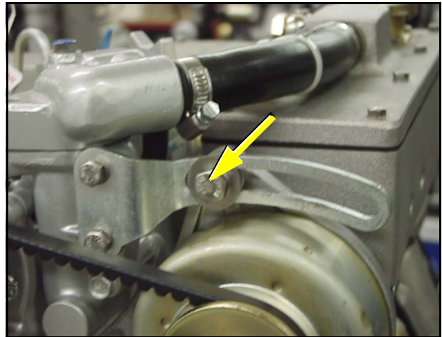
Fig. 10.15-1: Lichtmaschinen-Schraube
