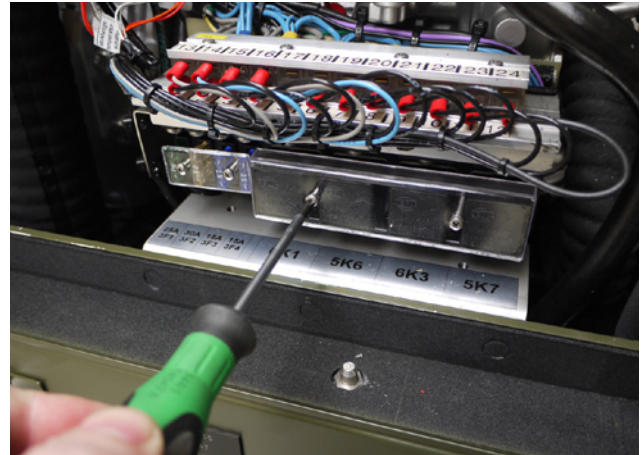
Fig. 10.13-1: Relais
