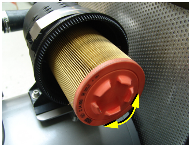
Fig. 10.9-5: Austausch Luftfilter
