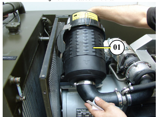
Fig. 10.9-2: Austausch Luftfilter
