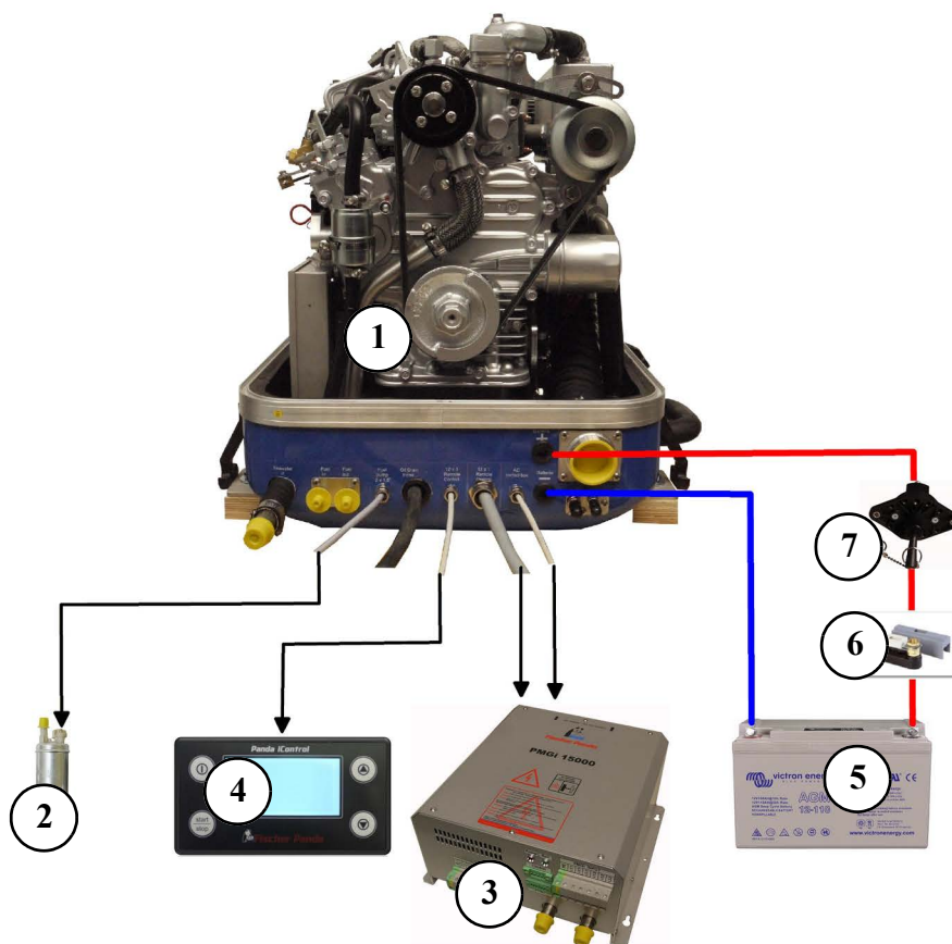
Fig. 8.12.0-1: Installationsschema Beispiel
