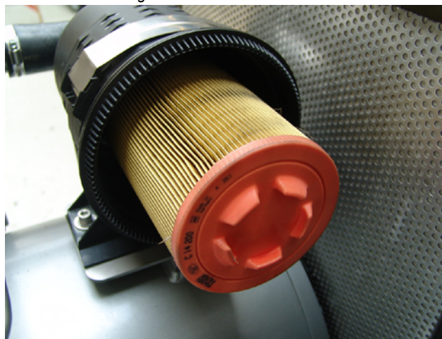
Fig. 10.9-6: Luftfilter reinigen
