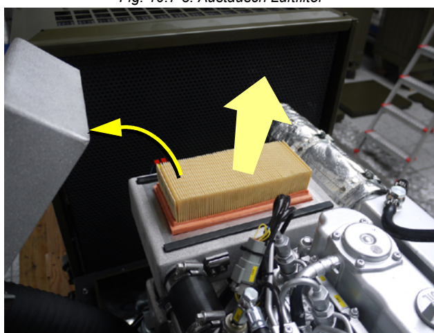
Fig. 10.7-3: Austausch Luftfilter
