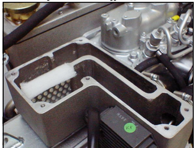
Fig. 10.8.0-2: Luftansauggehäuse offen
