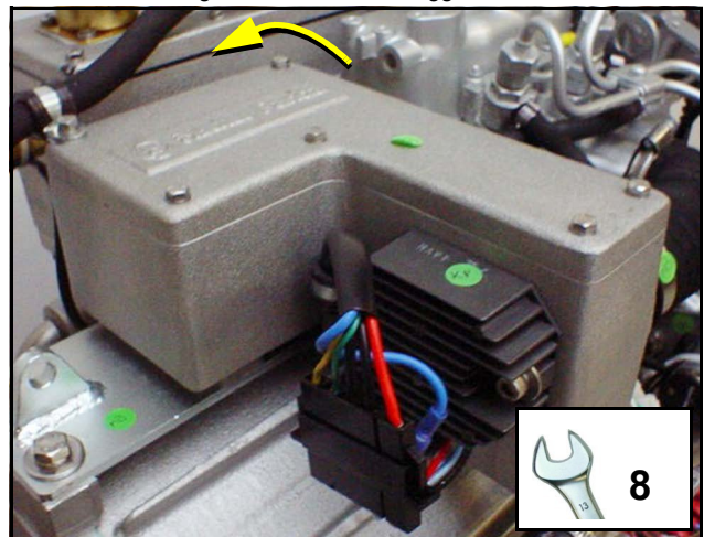
Fig. 10.8.0-1: Luftansauggehäuse
