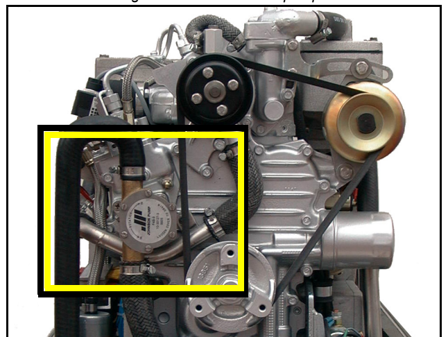
Fig. 10.5.3-3: Gehäuse Seewasserpumpe
