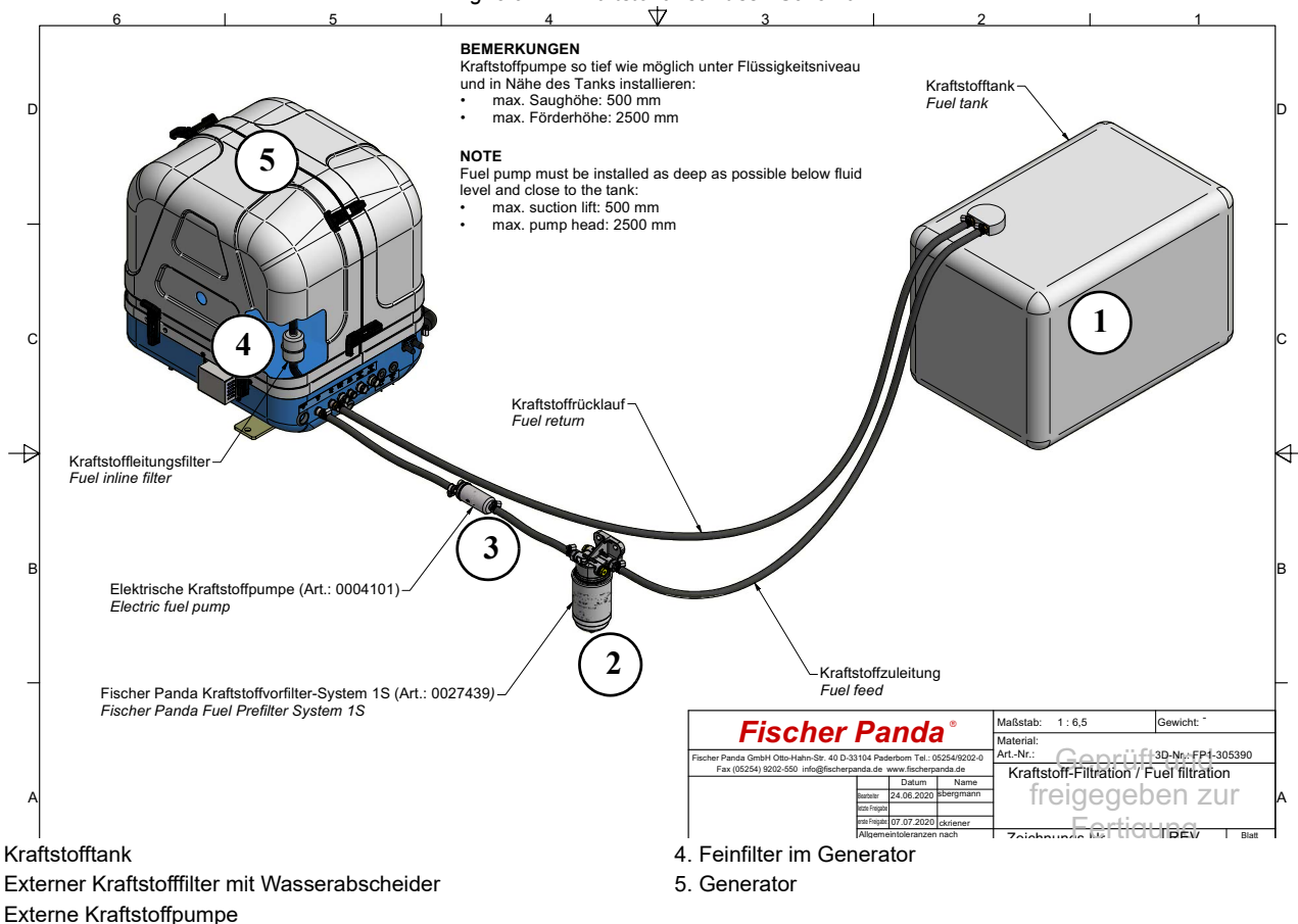
Fig. 8.9.1-2: Kraftstoffanschluss - Schema
