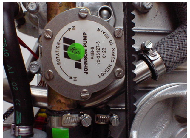
Fig. 10.5.3-3: Gehäuse Seewasserpumpe
