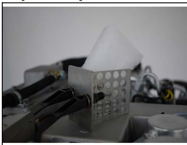
Fig. 10.8.1-4: Luftfiltergehäuse mit Schnellwechselhalter
