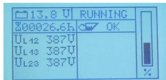
Fig. 15.3.3.4-4: Inverterseite Außenleiterspannungen
