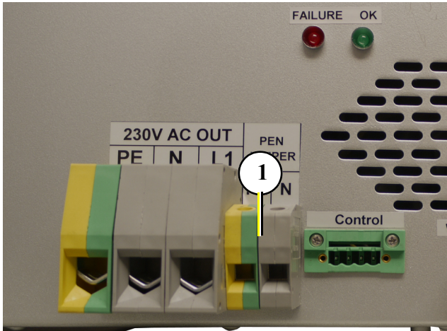
Fig. 13.11-1: PE-N Brücke
