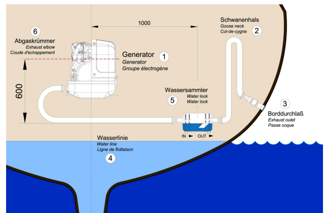
Fig. 8.6.3.2-3: Abgaswassersammler 1000 mm neben der Mittellinie des Generators
