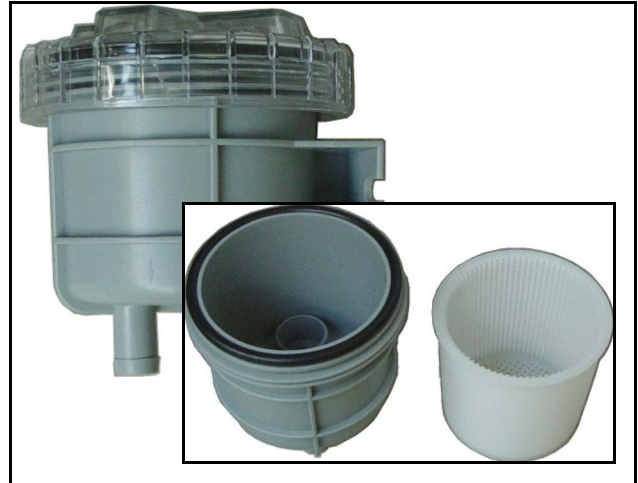
Fig. 10.5.1-1: Seewasserfilter
