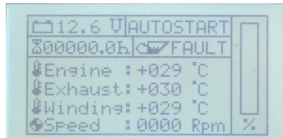
Fig. 15.4.6-7: Standard-Displayseite im Autostart-Modus
