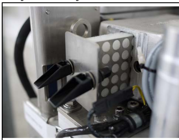
Fig. 10.8.1-3: Luftfiltergehäuse mit Schnellwechselhalter
