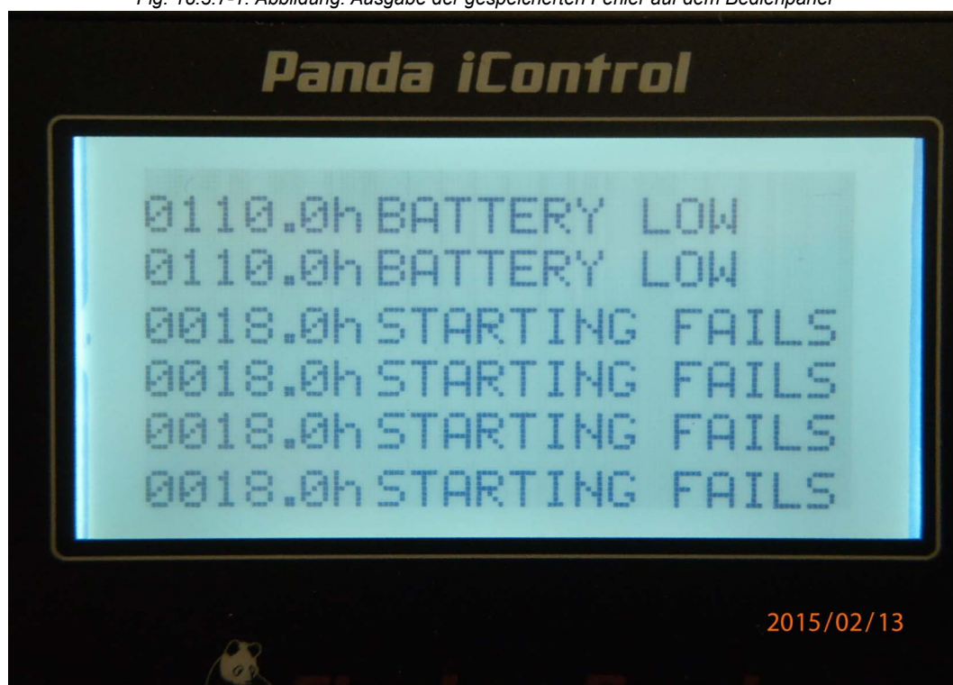
Fig. 18.3.7-1: Abbildung: Ausgabe der gespeicherten Fehler auf dem Bedienpanel
