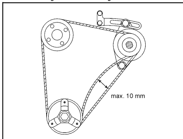
Fig. 10.15-4: Zeichnung Keilriemen
